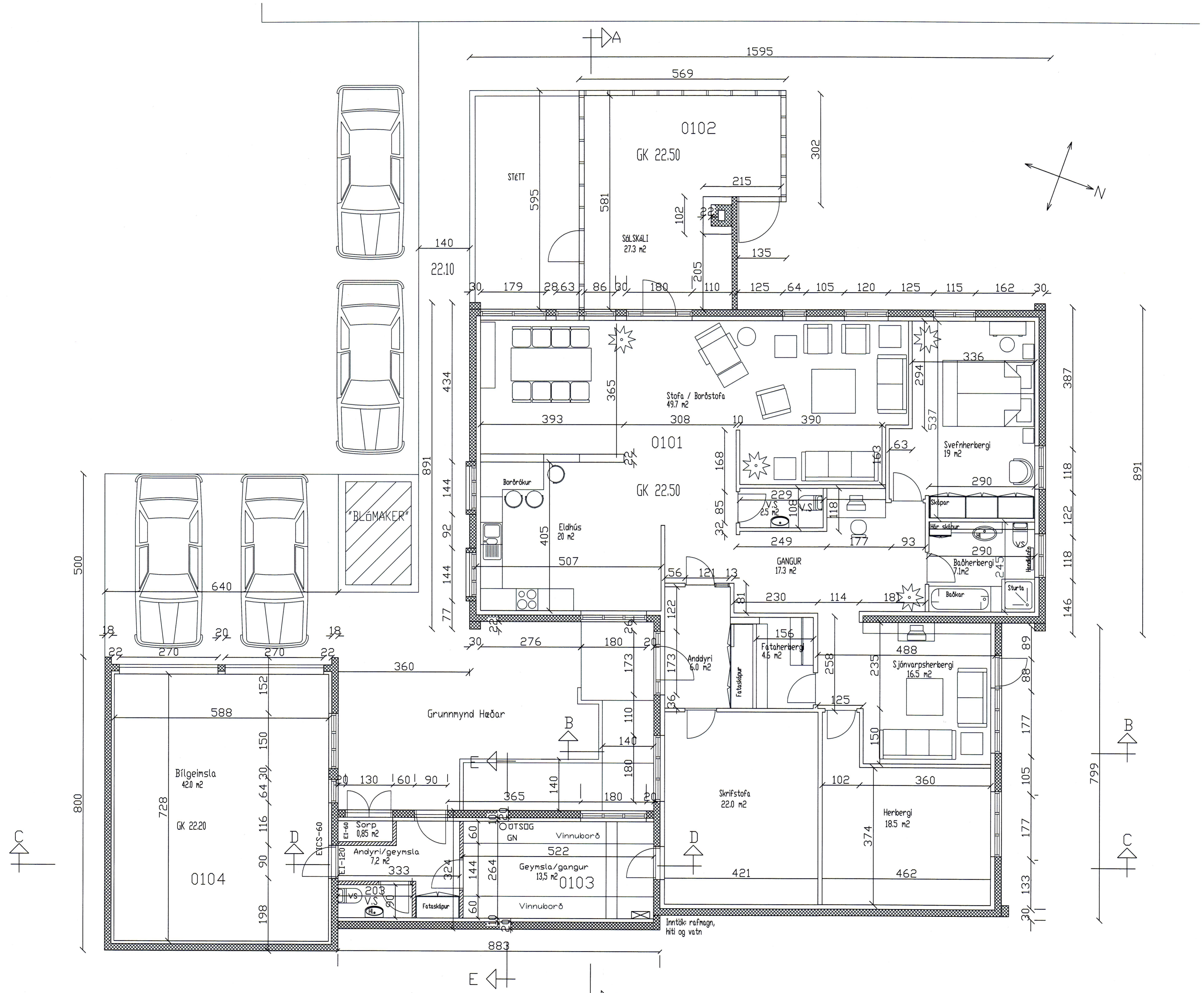
GRUNNMYND 1:50
