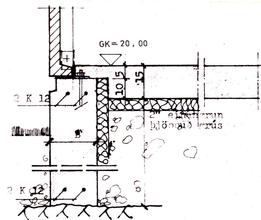
SNID Í SOKKLA: M 1:10.
