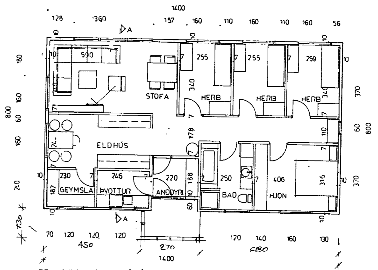
GRUNNMYND 1:100
