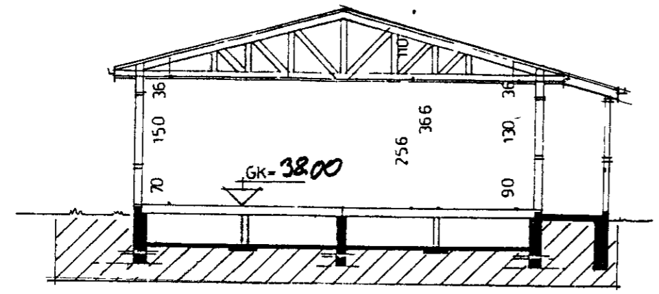
SNID A-A 1:100
