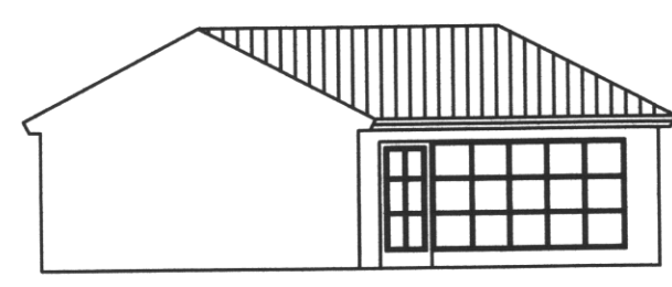
ÚTLIT-VESTUR mkv: 1:100
