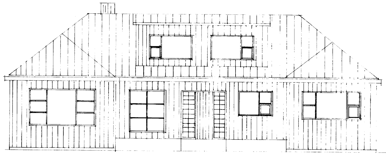
SUÐURHLÍÐ M=1:100
