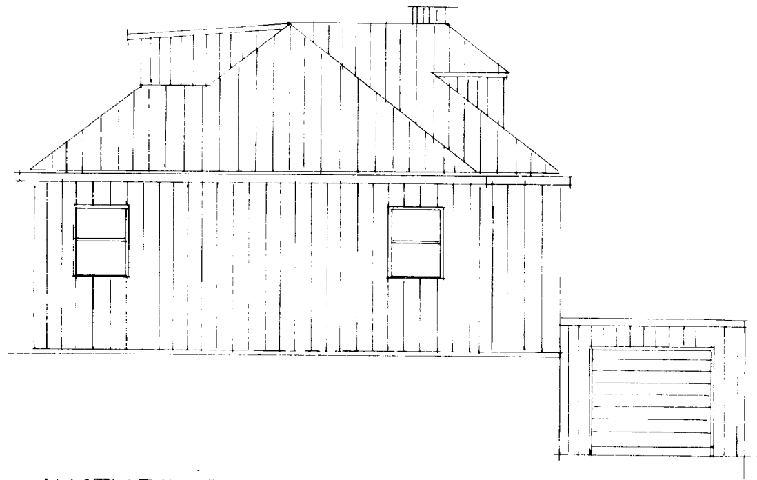
AUSTURHLÍÐ M=1:100
