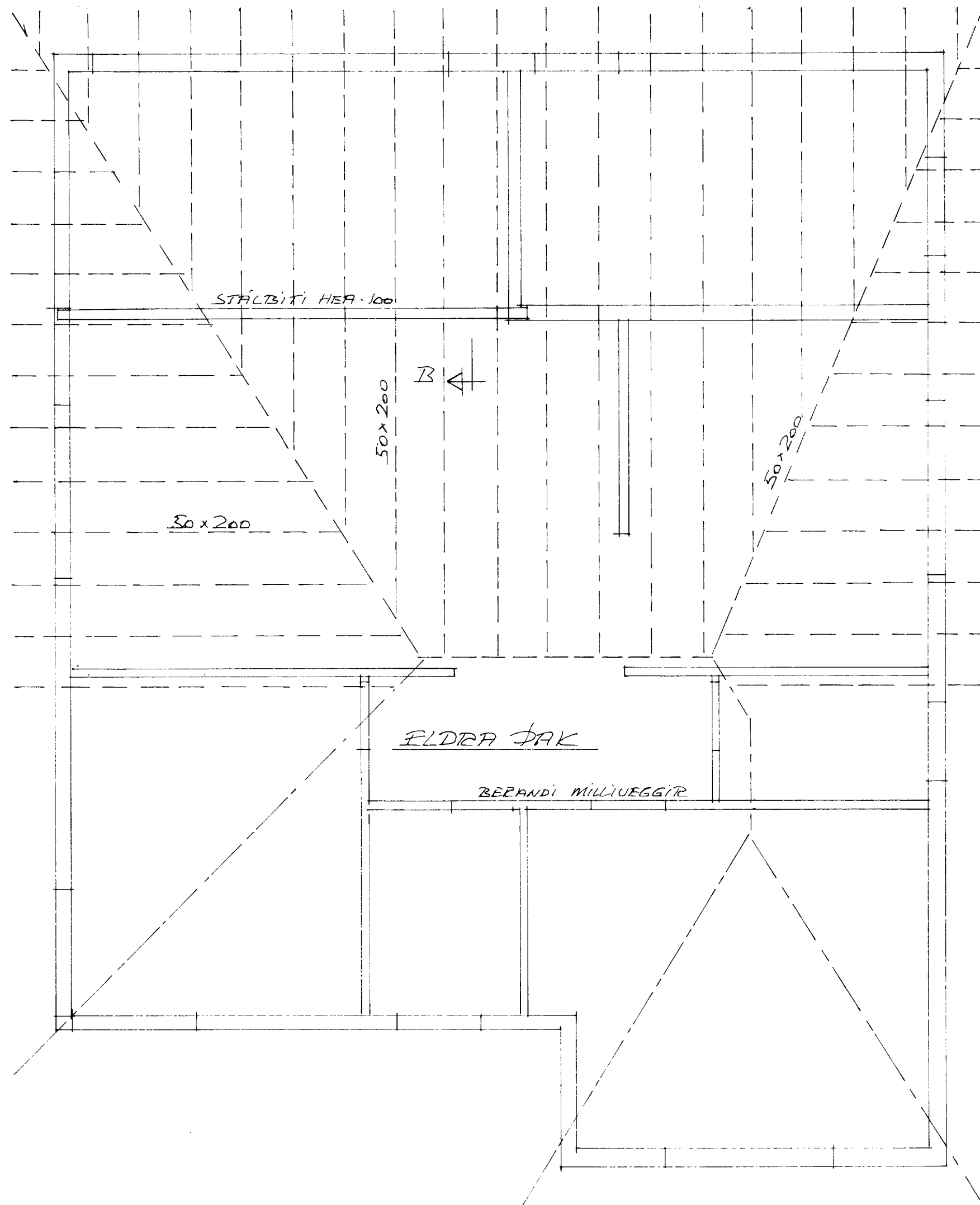
GRUNNMUND SPERBLUR 1:50
