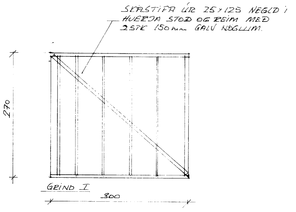
GRUNNMÝND GRINDAR 1:50
