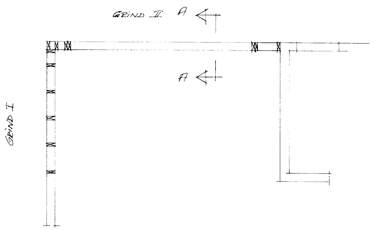
GRUNNMÝND GRINDAR 1:50
