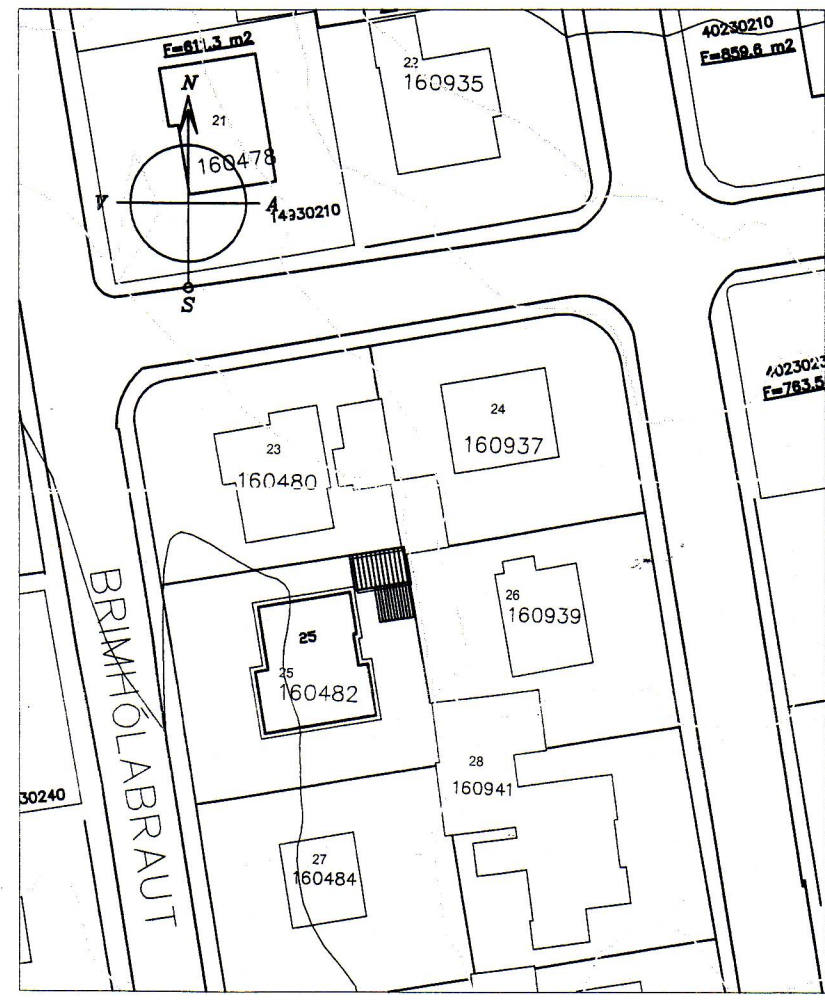
AFSTÖÐUMYND 1:500
