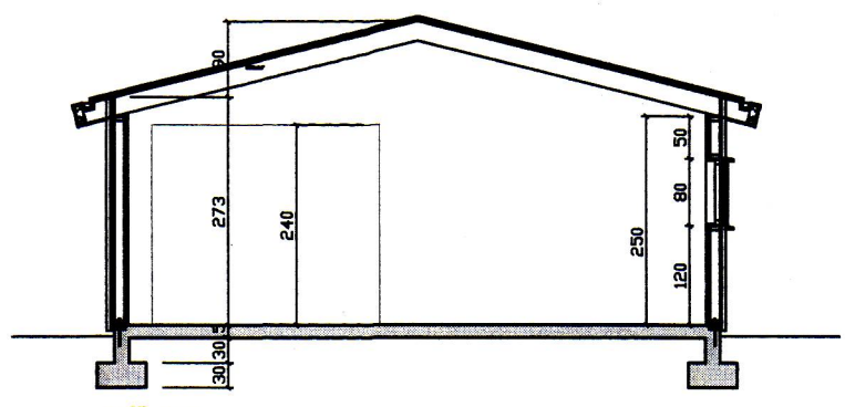
SNID A-A
