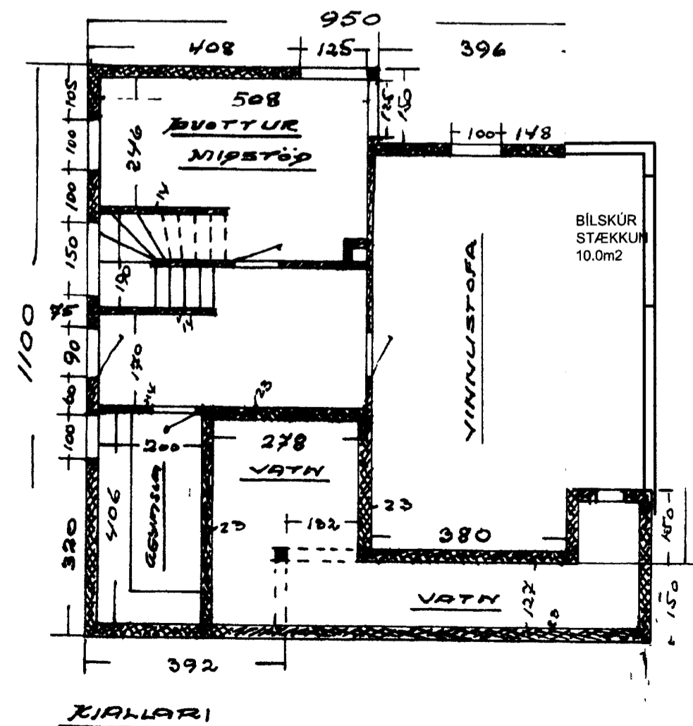
TVALARI
