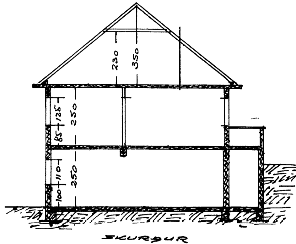
SKURÐUR
