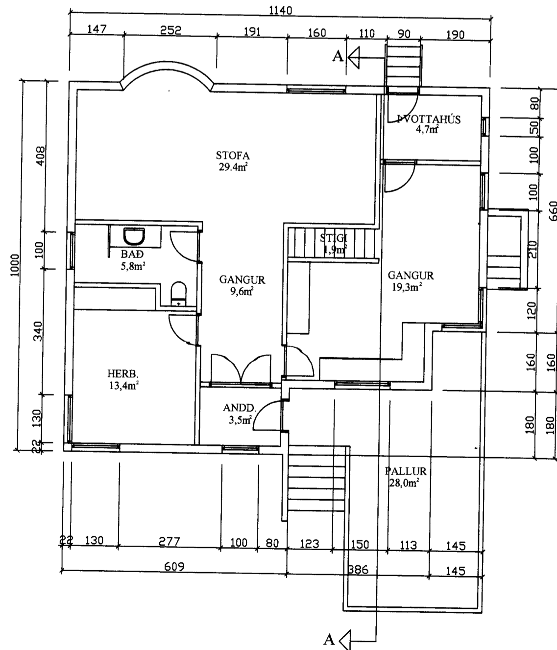
GRUNNMYND 1. HÆÐ
