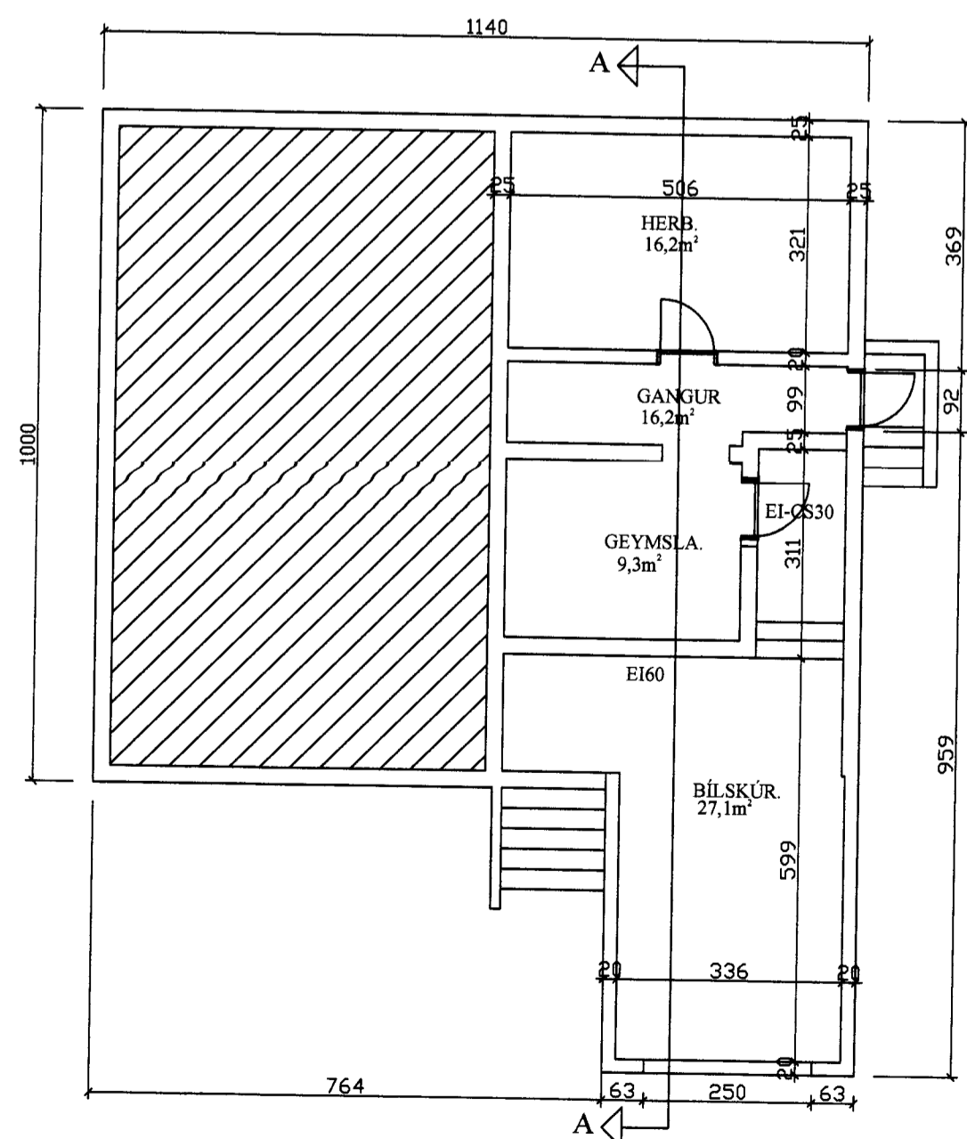
GRUNNMYND KJALLARI
