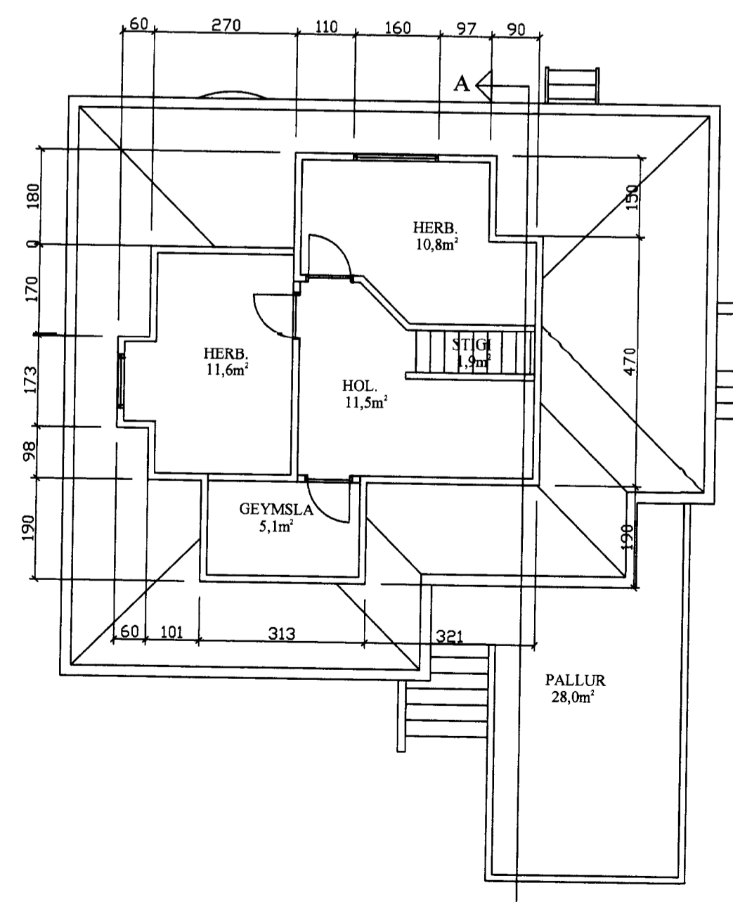
GRUNNMYND 2. HÆÐ
