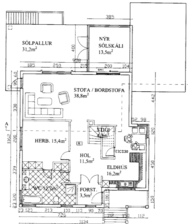
1 HÆÐ
