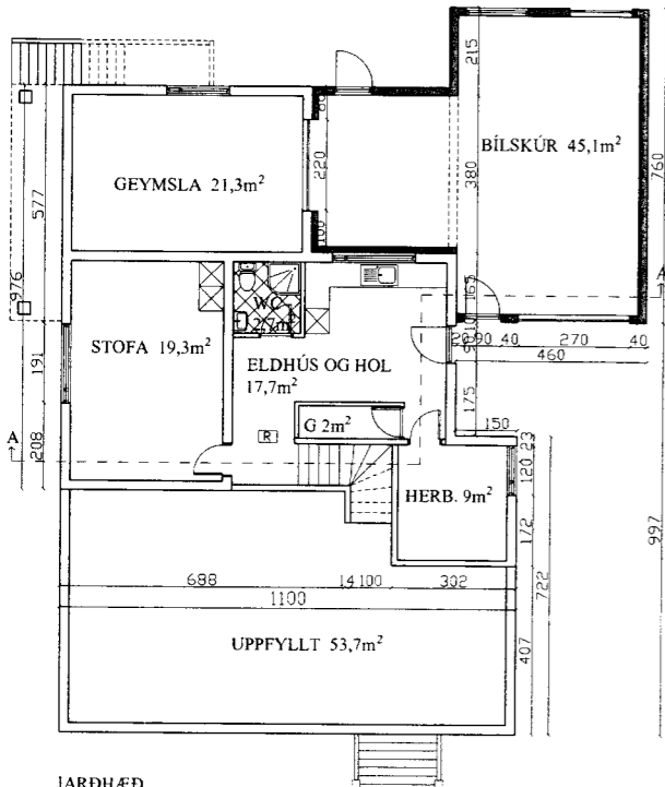
JARDHÆÐ
