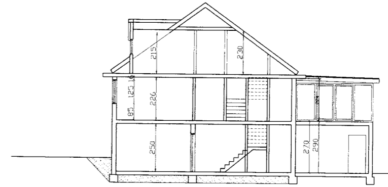
SNIÐ A:A
