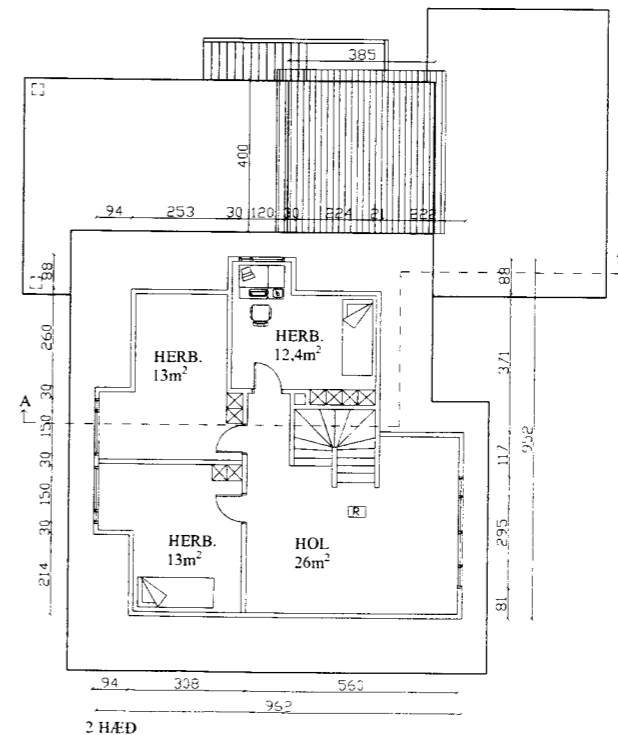
2 HÆÐ
