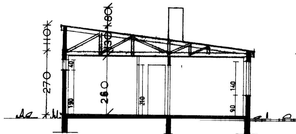
SNEIÐING A-A
