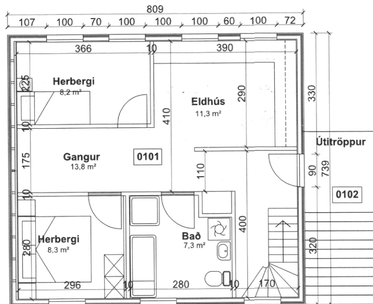
Grunnmynd, 1. hæð M=1:100
