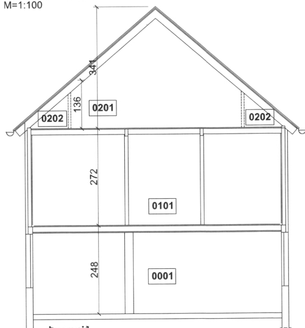
Þversnið M=1:100
