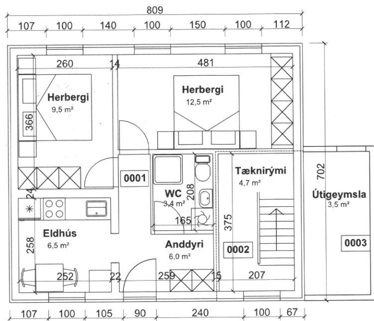
Grunnmynd, Kjallari M=1:100
