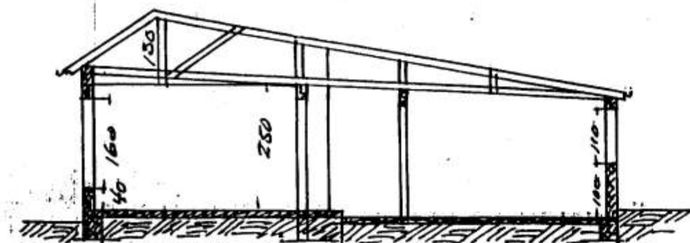
SKURÐUR
