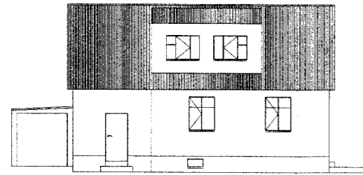
ÚTLIT NORÐUR
