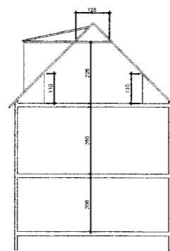
SNID A-A
