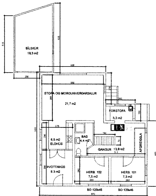
GRUNNMYND 1.HÆÐ
