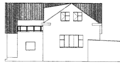
ÚTLIT SUÐUR
