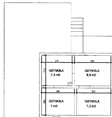
GRUNNMYND KJALLARI
