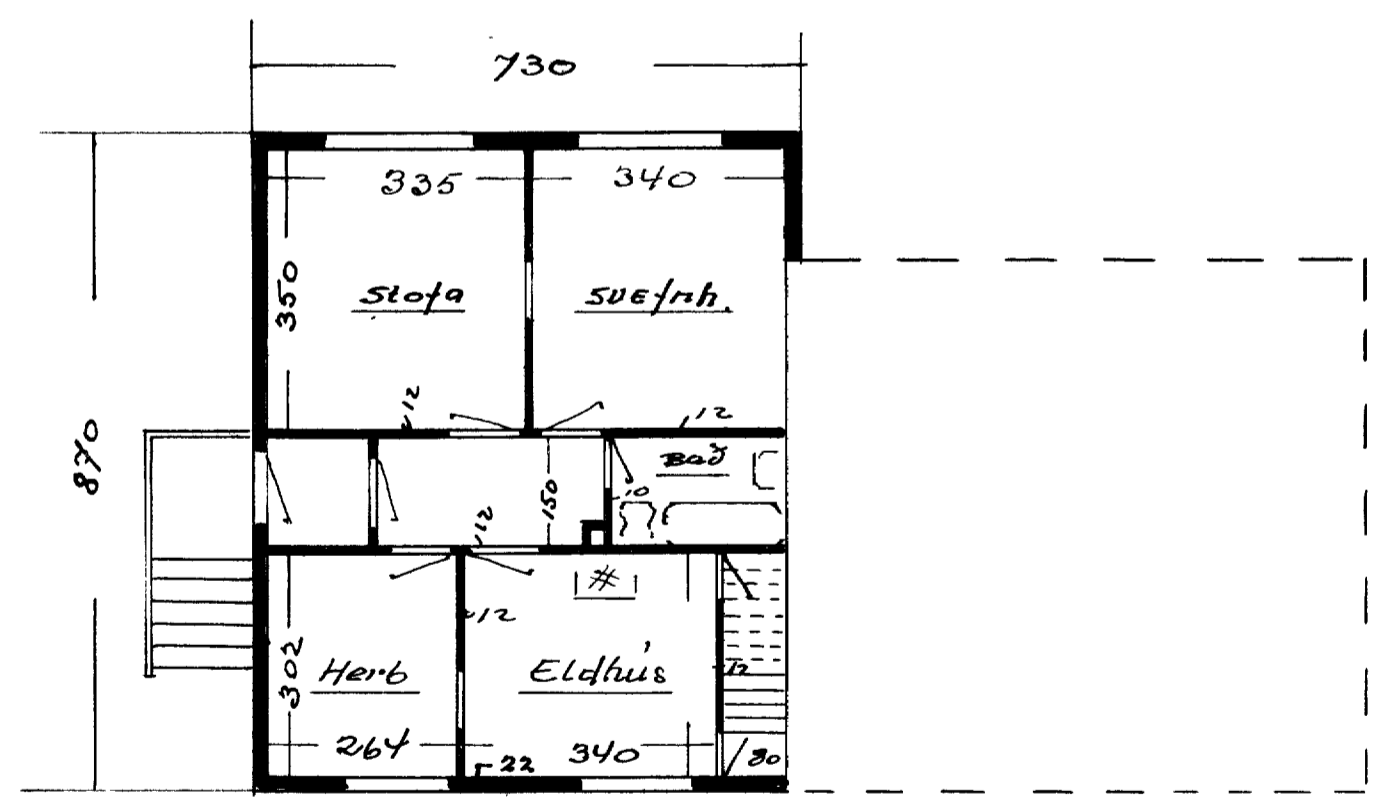
1. HÆÐ
