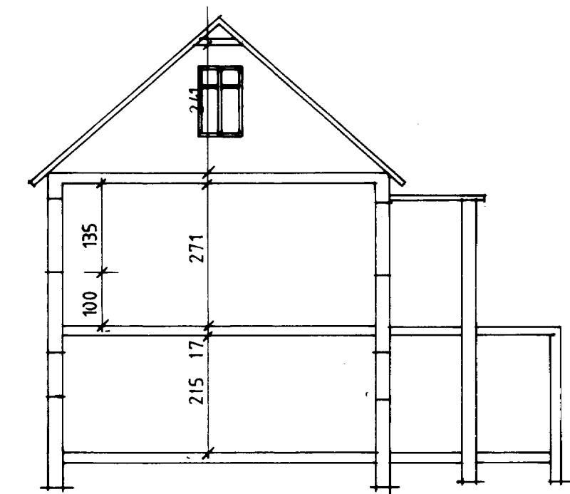
SNIÐ A-A
