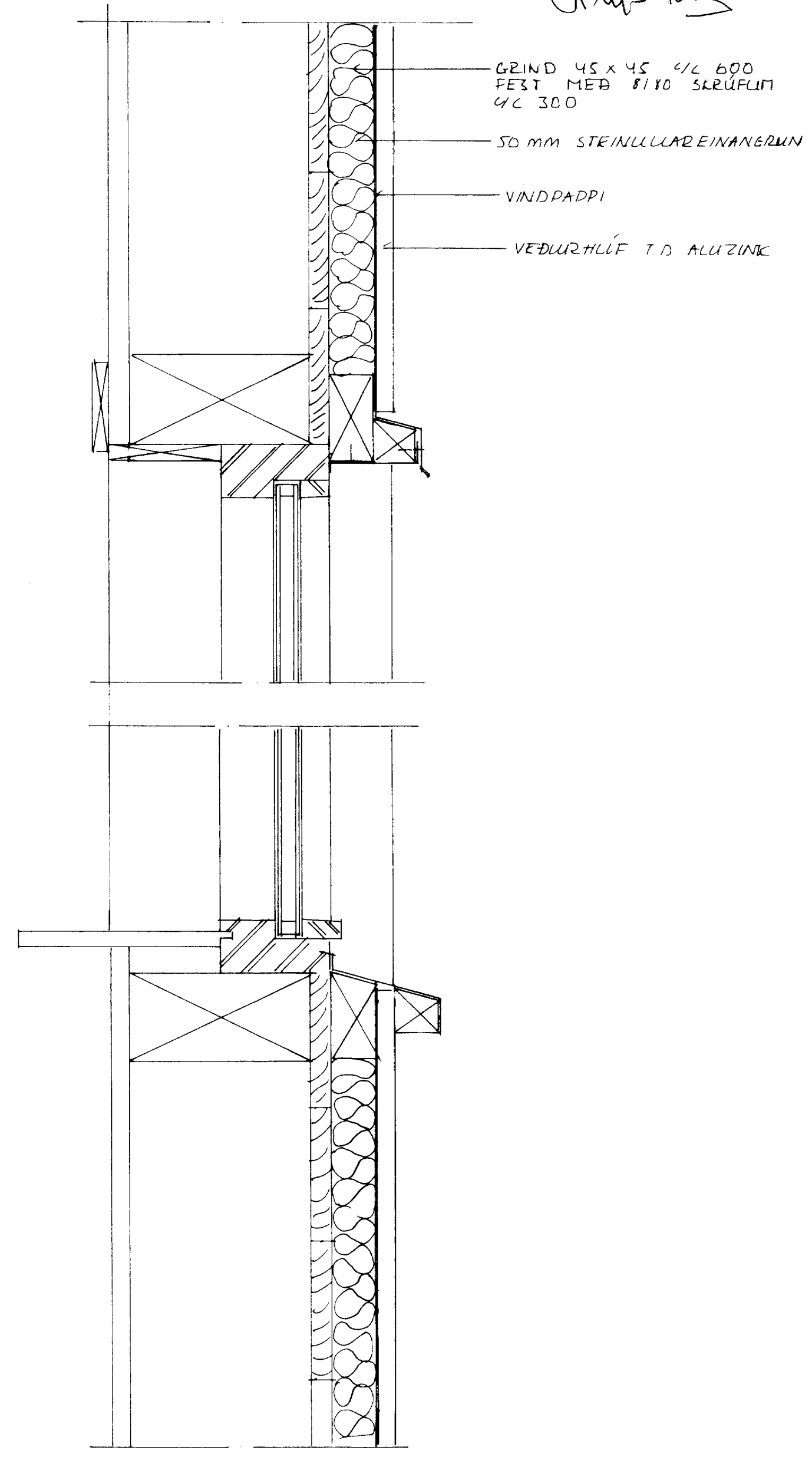
LÓDRÉTT SNID Í TRÉÚTVEGG MKV 1:5
