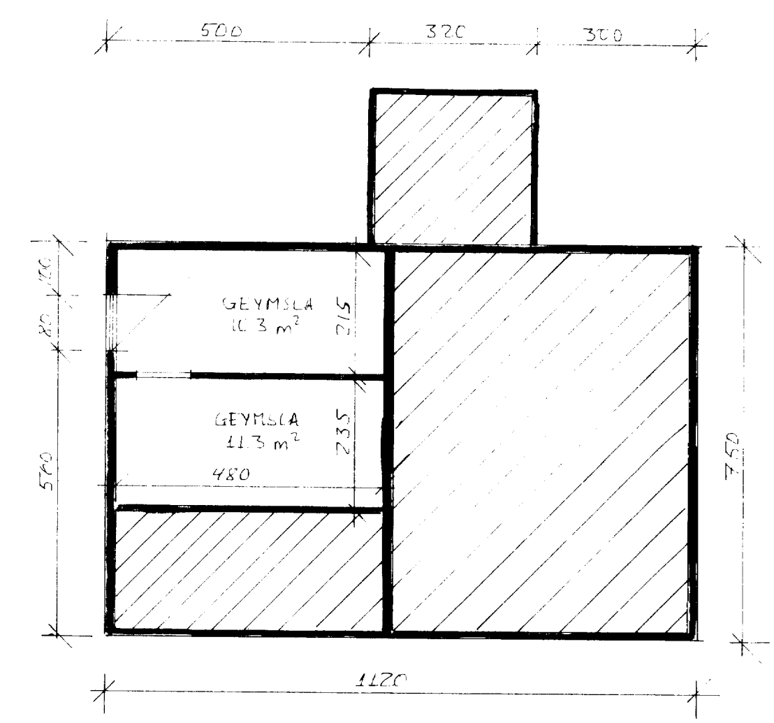
GRUNNMYND KJALLARI MKV 1:100
