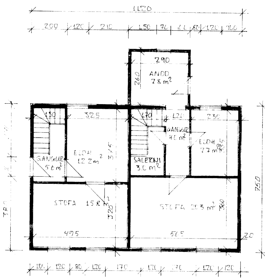
GRUNNMYND 1 HÆÐ MKV 1:100
