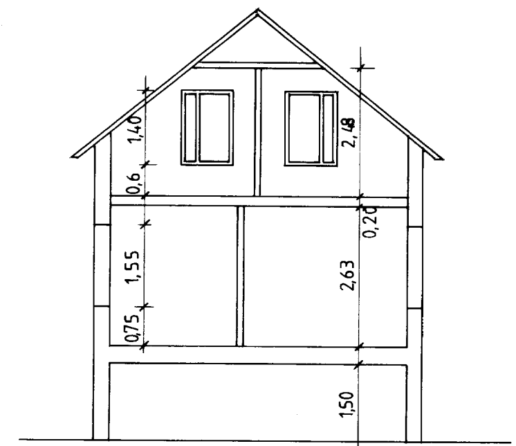
SNIB a-a
