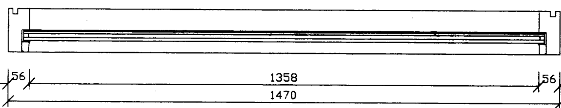
1 STK. RIS M=1:20
