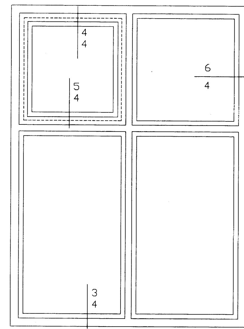
2 STK. KJALLARA M=1:20
