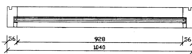
3 STK. 1. HÆÐ M=1:20
