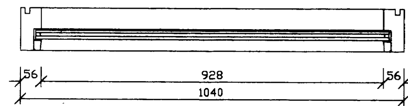
2 STK. 1. HÆÐ M=1:20
