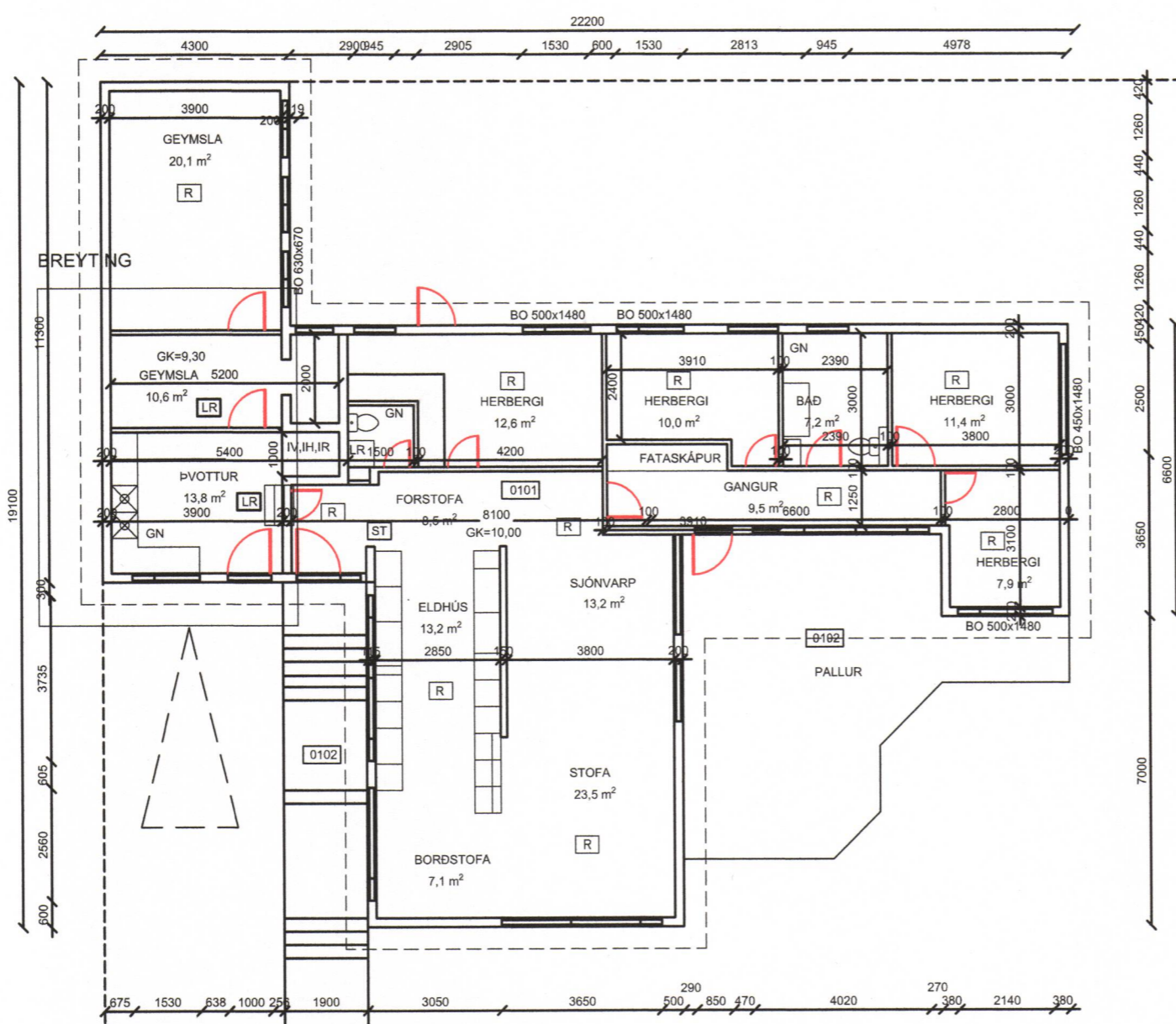
GRUNNMYND 1:100
