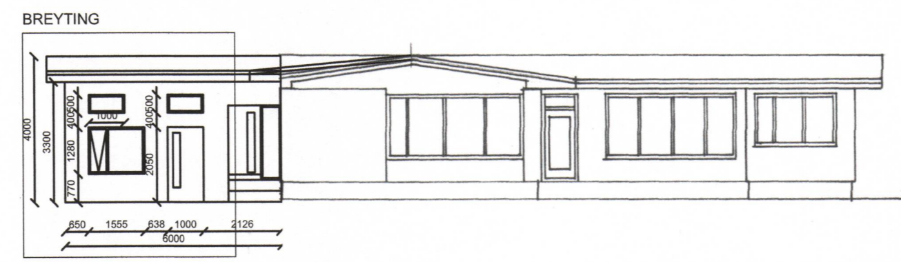
ÁSÝND VESTUR 1:100
