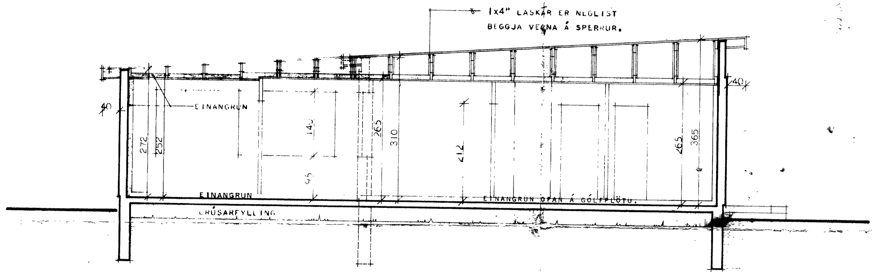
SNEIÐING A-A
