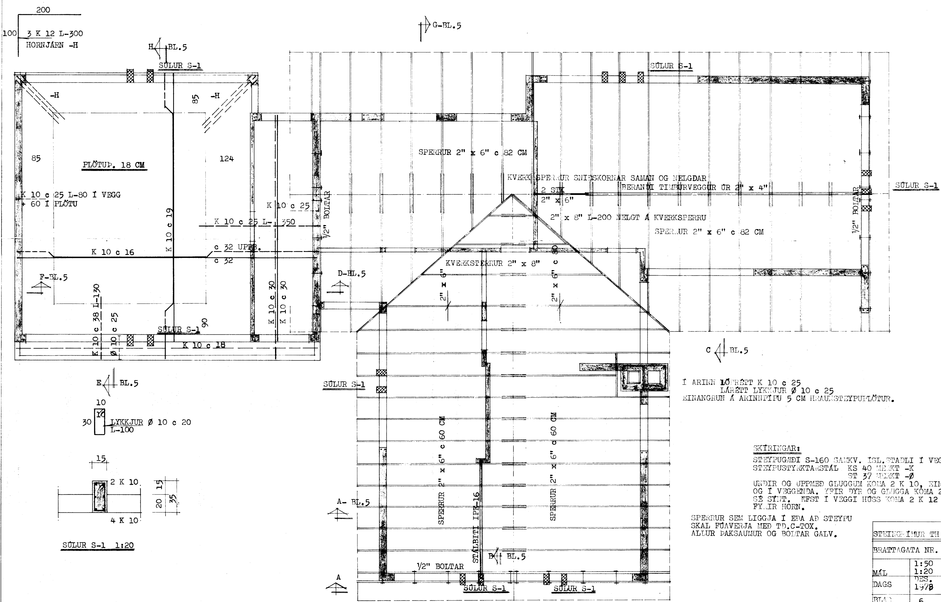
-A 1:50
