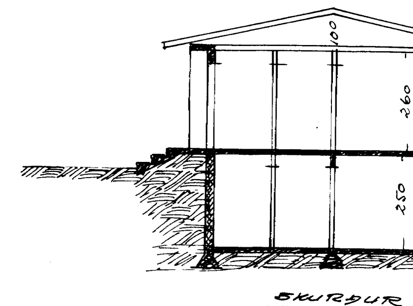
SKURÐUR
