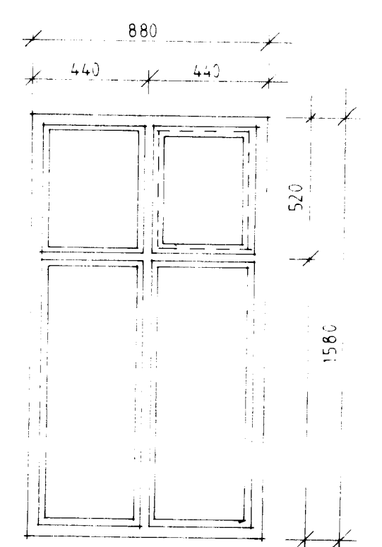
GLUGGAR 26 STK.
