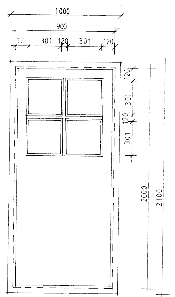
ÚTIHURÐIR 5 STK.
