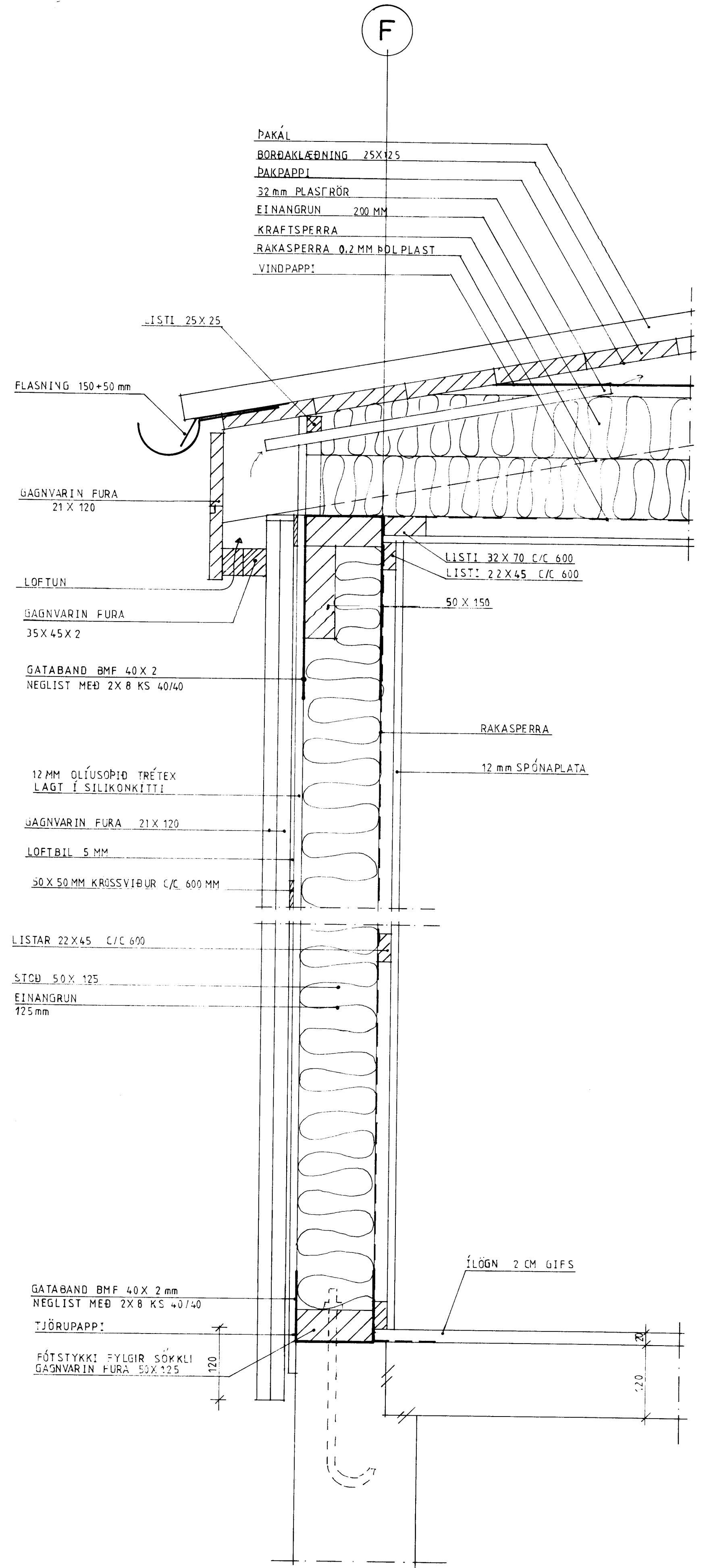
SNÍÐ Í ÚTVEGG 1:5
