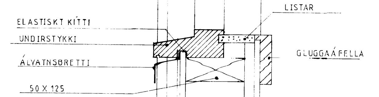
SNÍÐ Í GLUGGA 1:5
