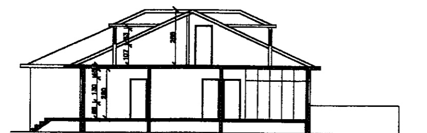
SKURÐUR M=1:100
