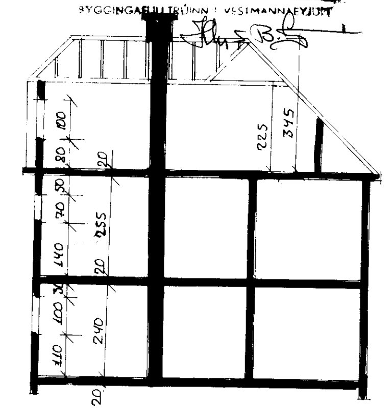
SNÍÐ Í BÚÐARHÚS
