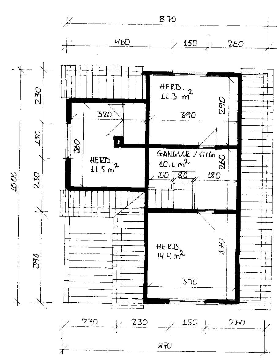
GRUNNMÝND RISTHÆÐ
