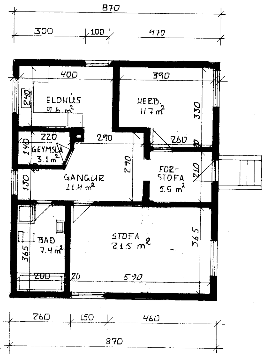
GRUNNMÝND KJALLARA
