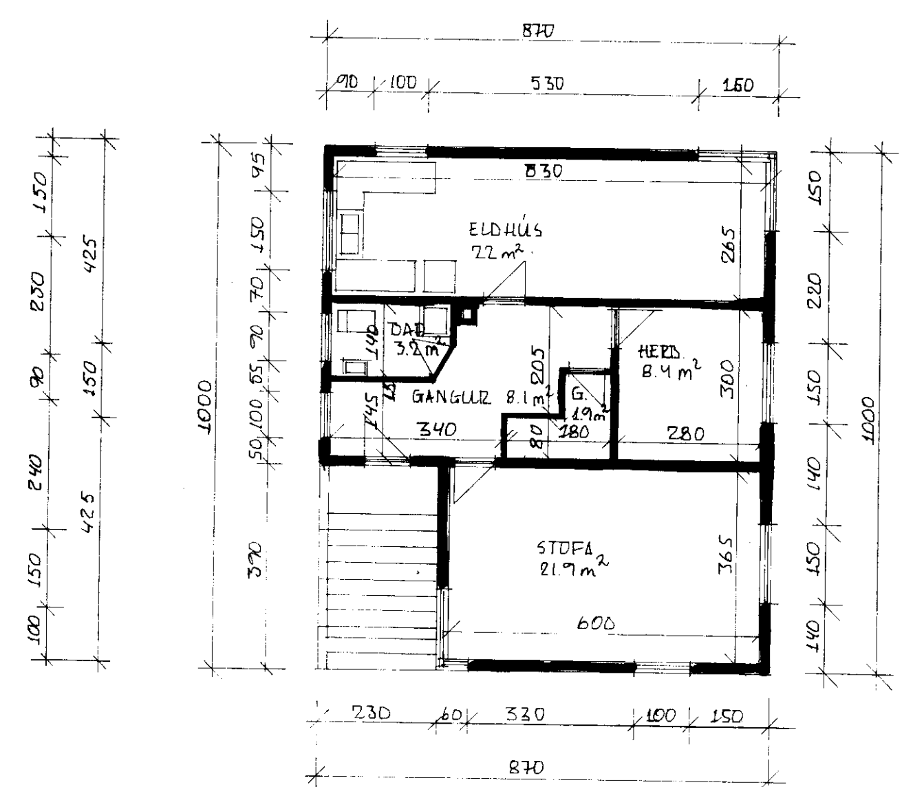
GRUNNMÝND MIÐHÆÐ
