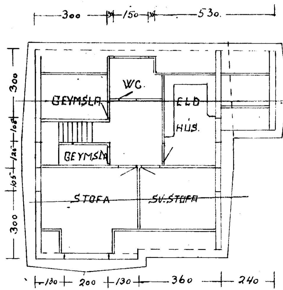
RISHÆÐ.
