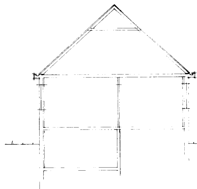
SNÍÐ B-B
