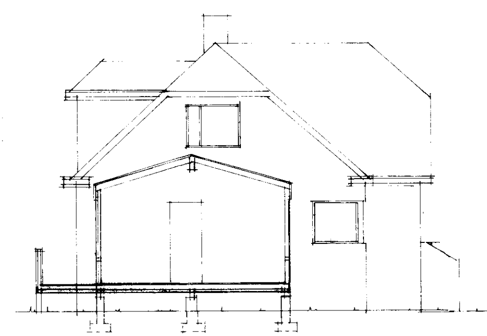
SNÍÐ C-C
