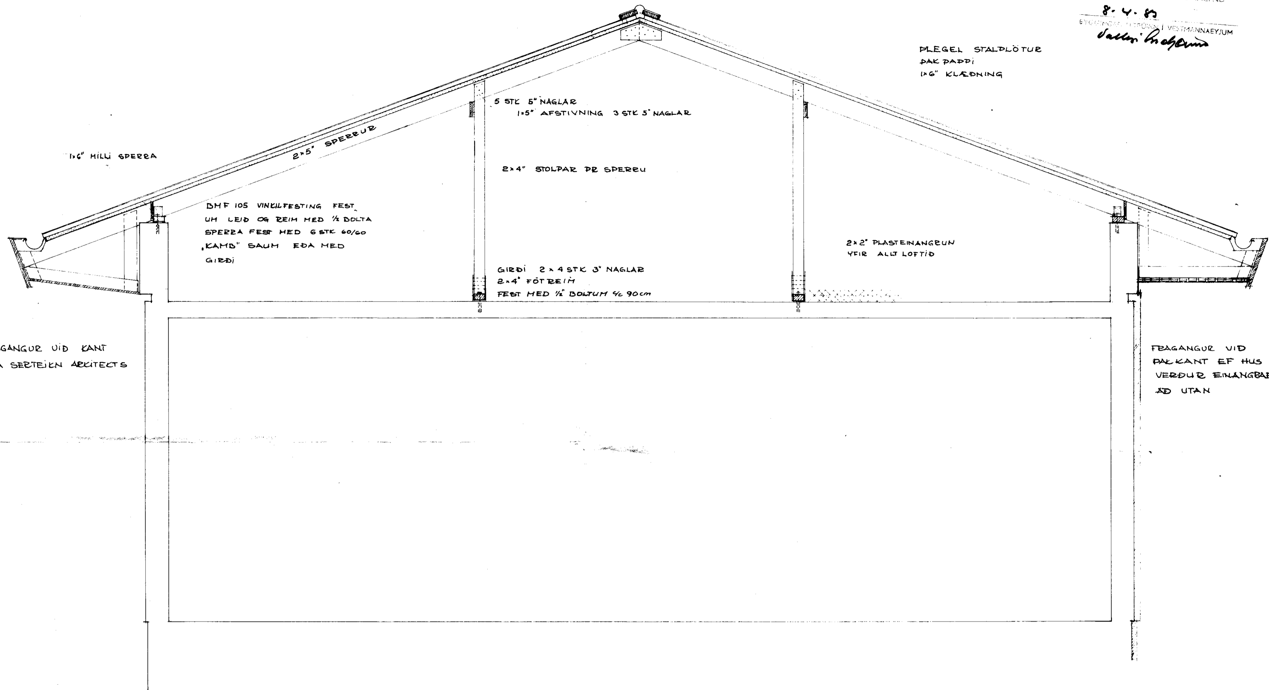
ÞVERSNIÐ 1:20
