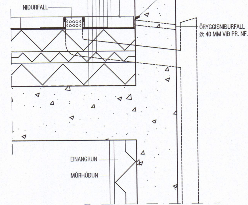
FRÁGANGUR ÞAKS VIÐ NIÐURFALL AF SVÖLUM
