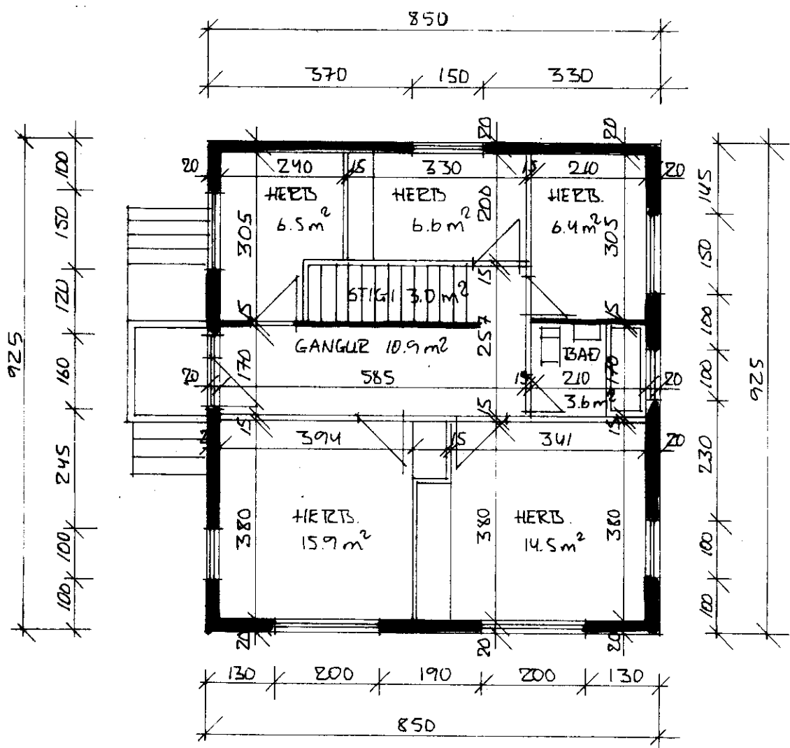
GRUNNMYND 2. HÆÐ M=1:100
