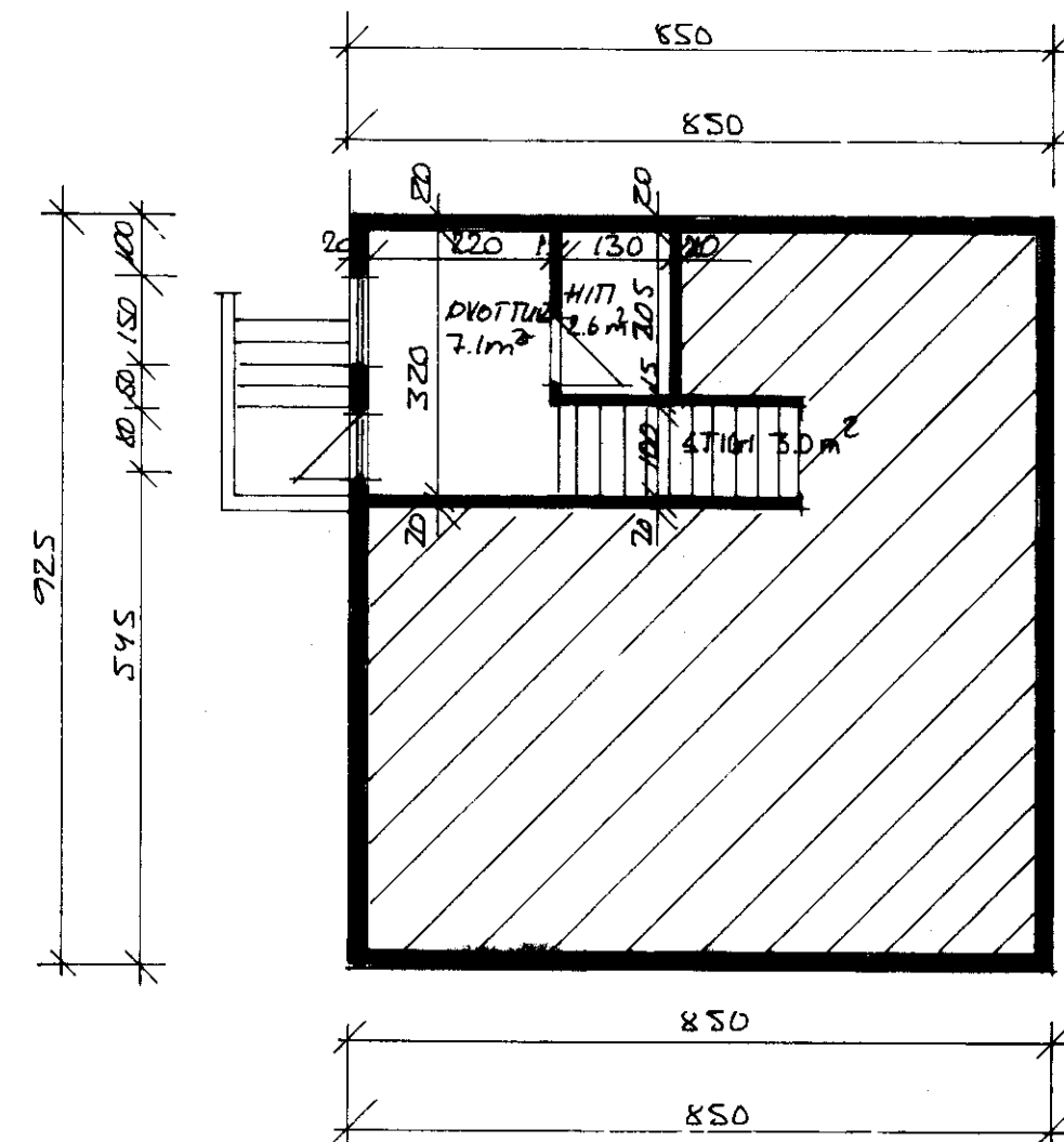
KJALLARI M=1:100
