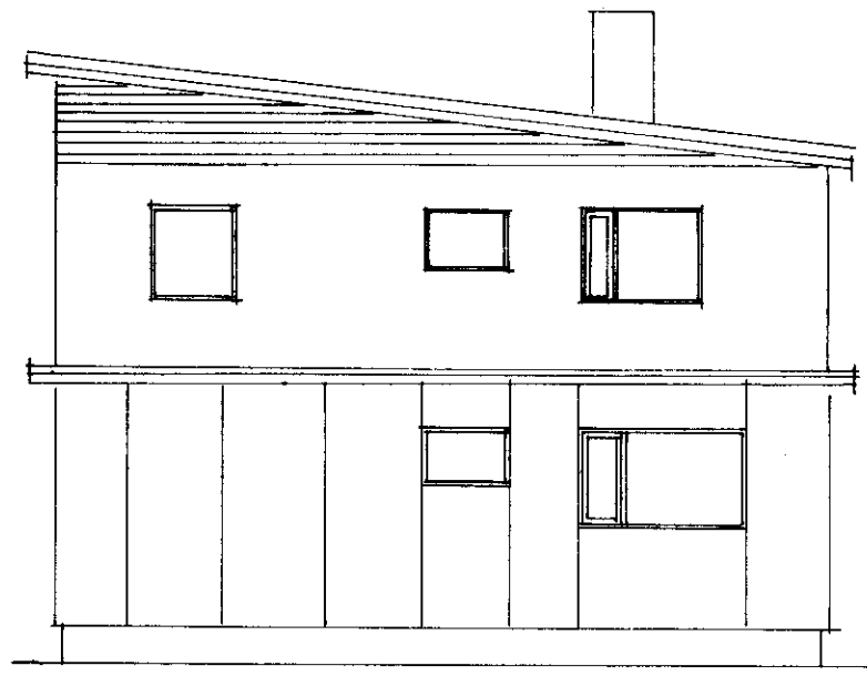
AUSTURHLID M=1:100
