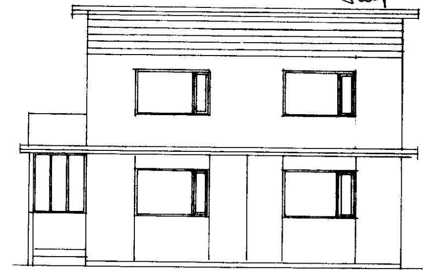
SUÐURHLID M=1:100
