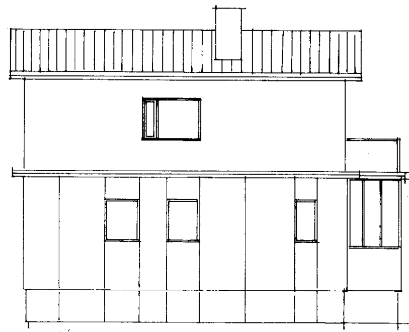
NORÐURHLID M=1:100
