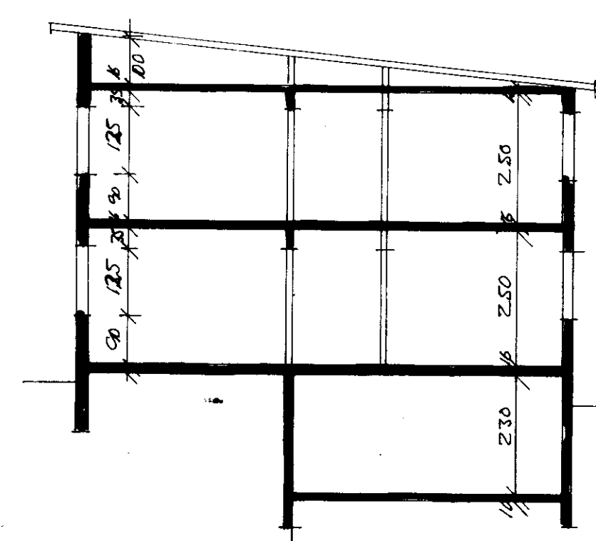
SKURÐUR M=1:100
