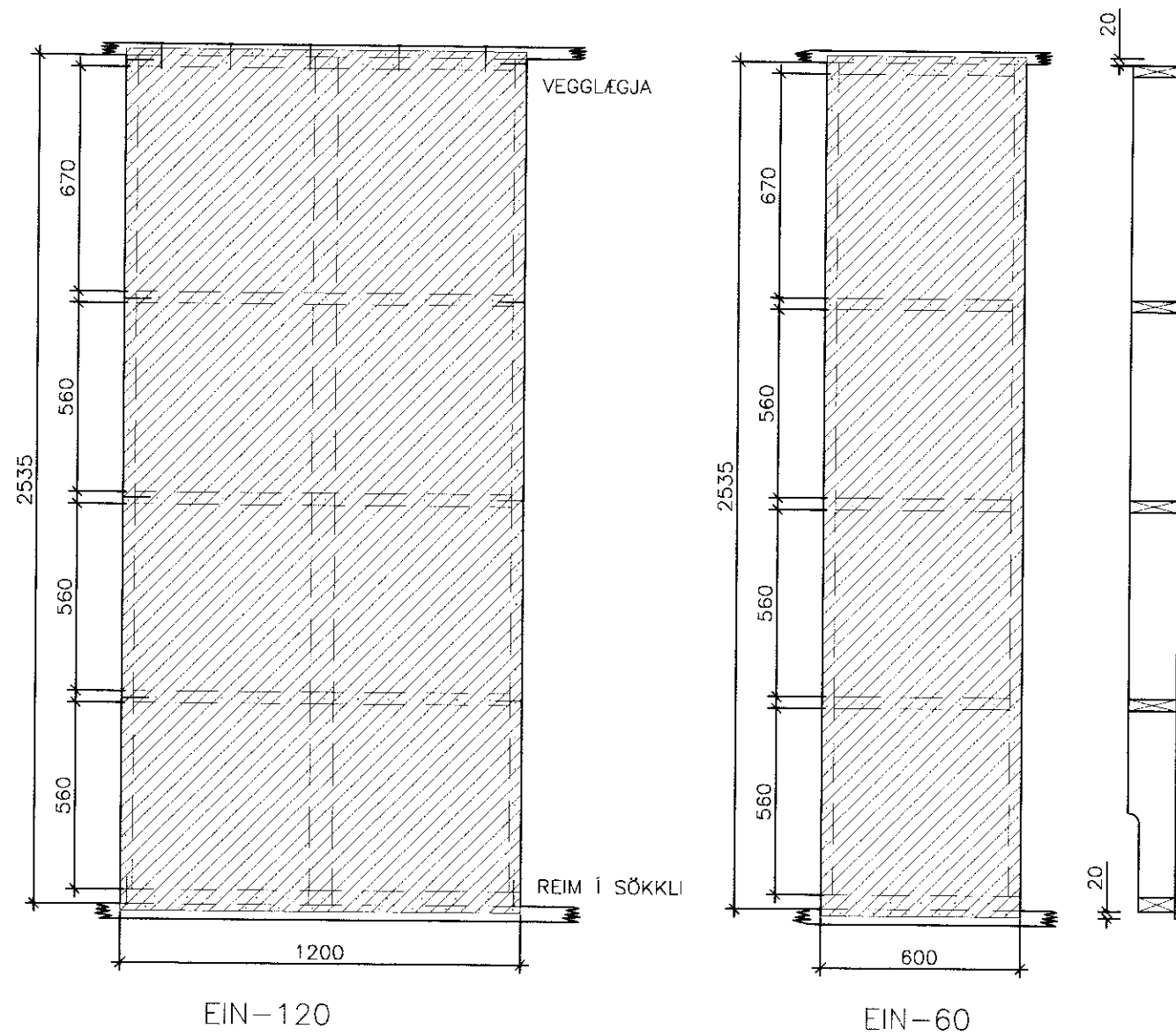
KROSSVÍÐARSTÍFINGAR Mkv. 1:20
