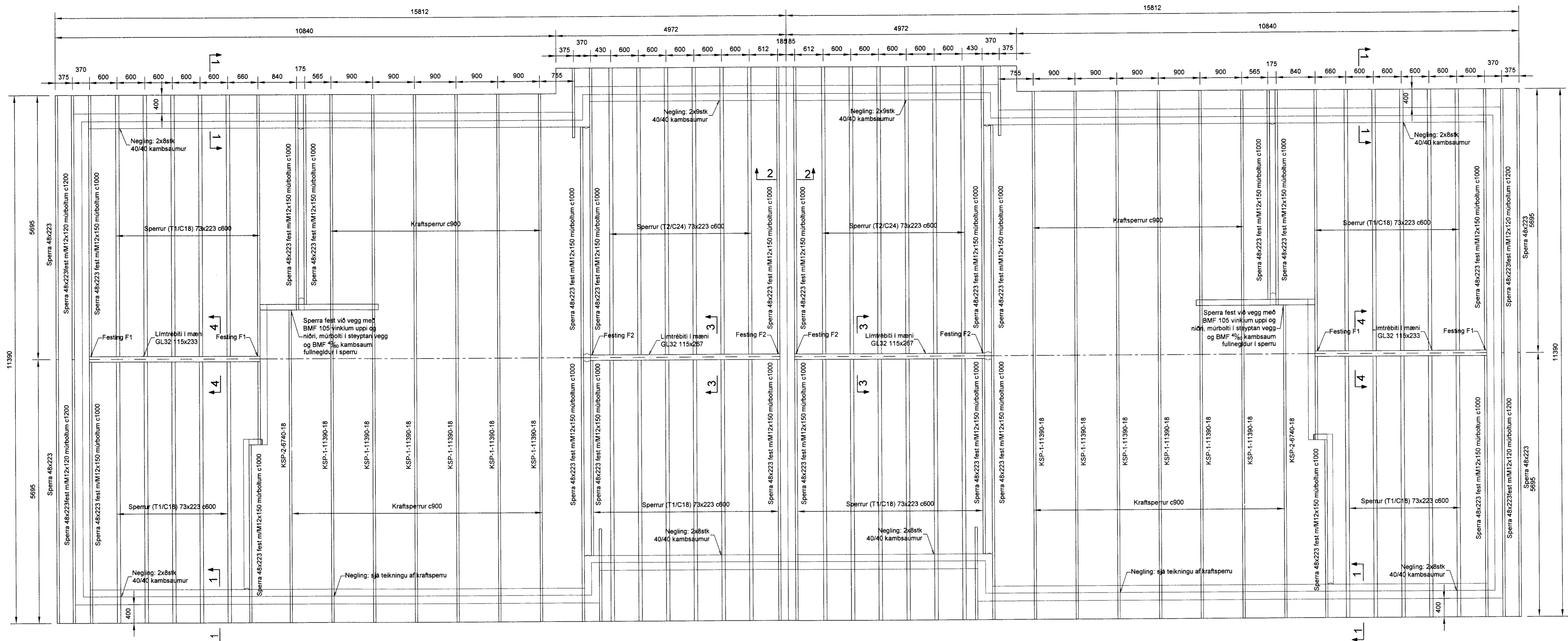
Grunnmynd þakvirkis 1:50
