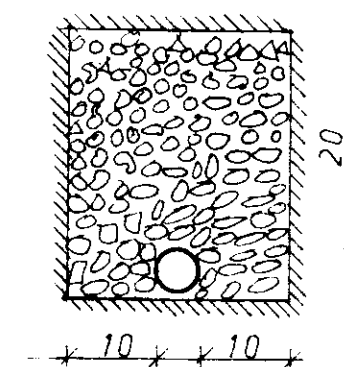
JARÐVATNSLÖGN PVERSNID 1:10
