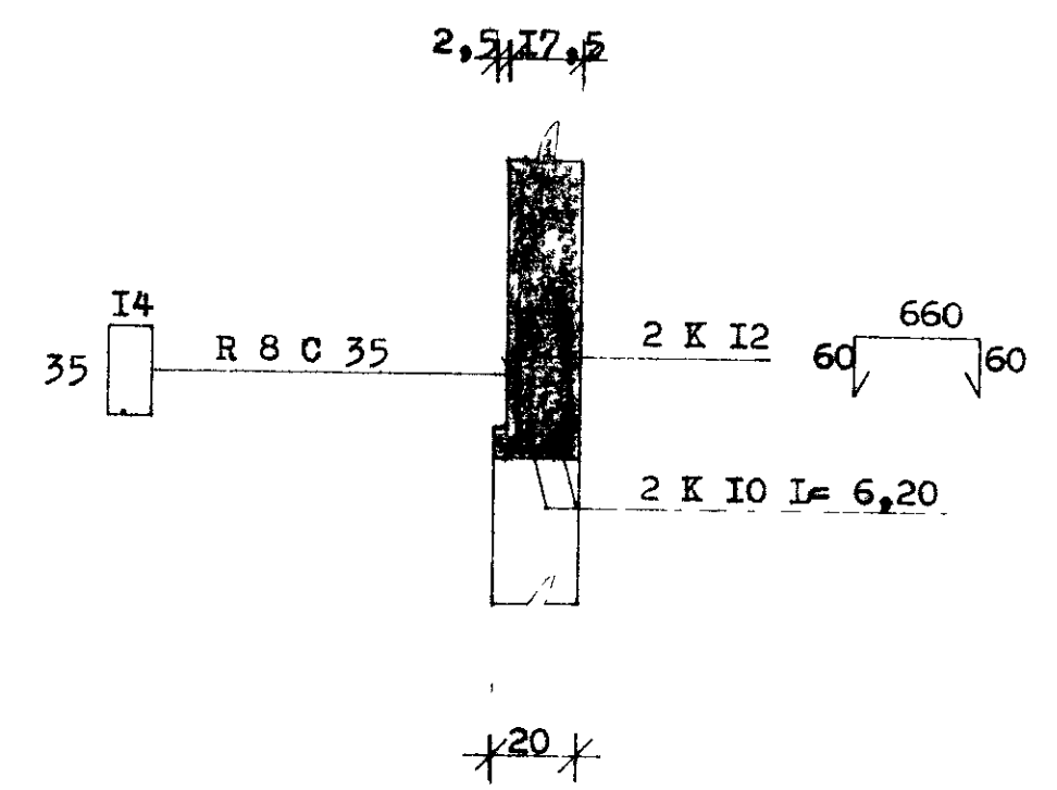
SNID B - B 1:20
