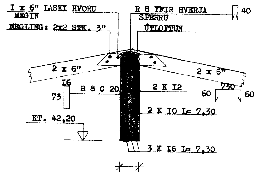
SNID B - B 1:20
