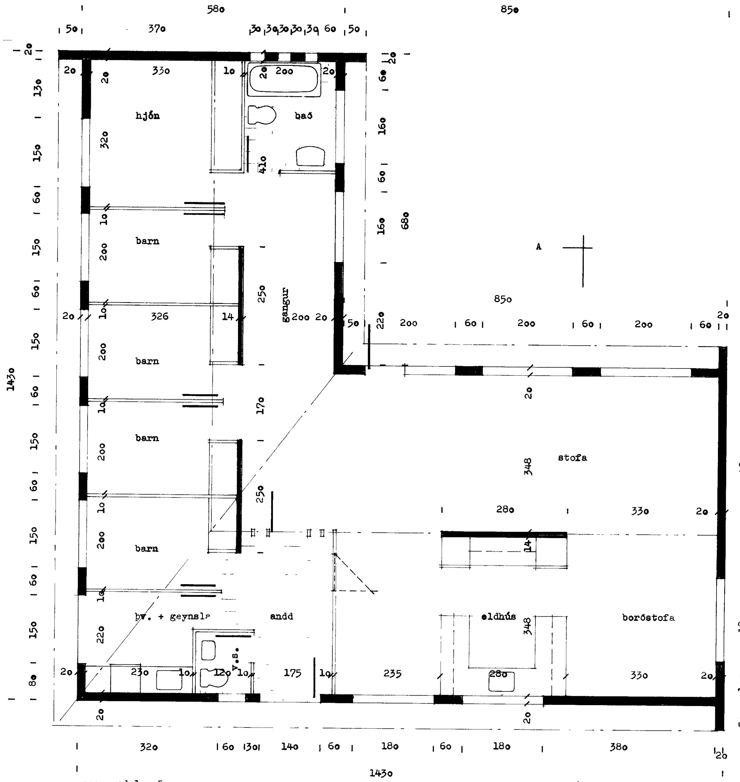
grunnmynd 1 : 50
