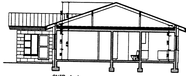
SNÍÐ A-A
