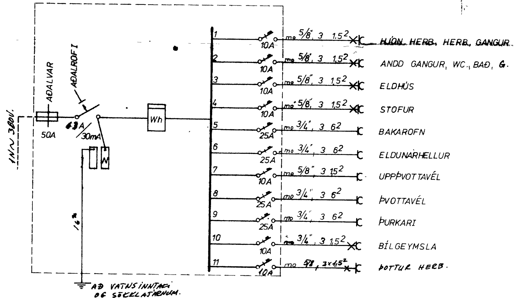
TENGYMYND
