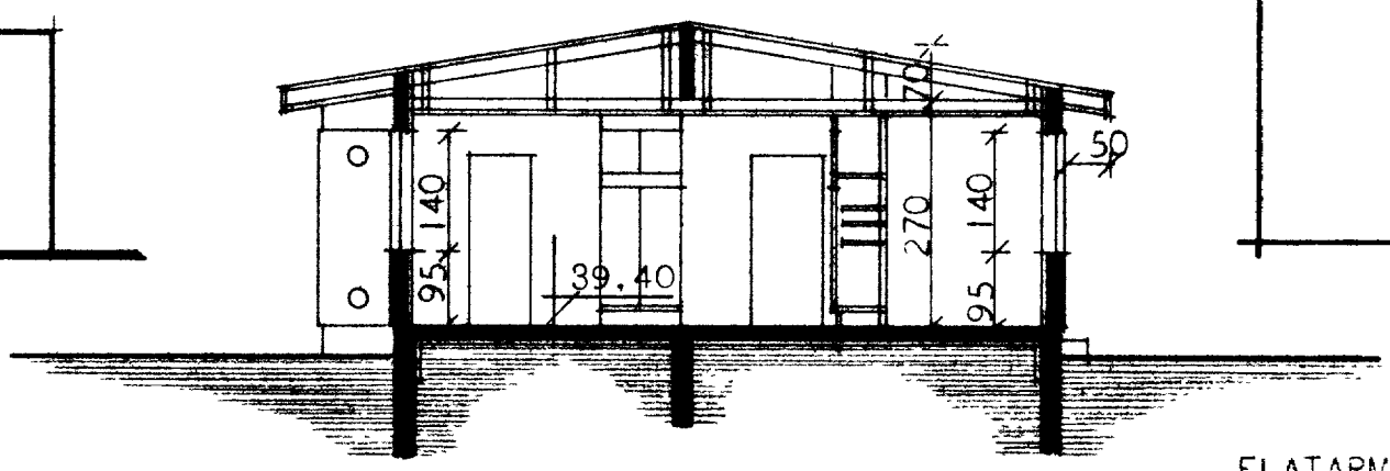
SNEIDING A-A
