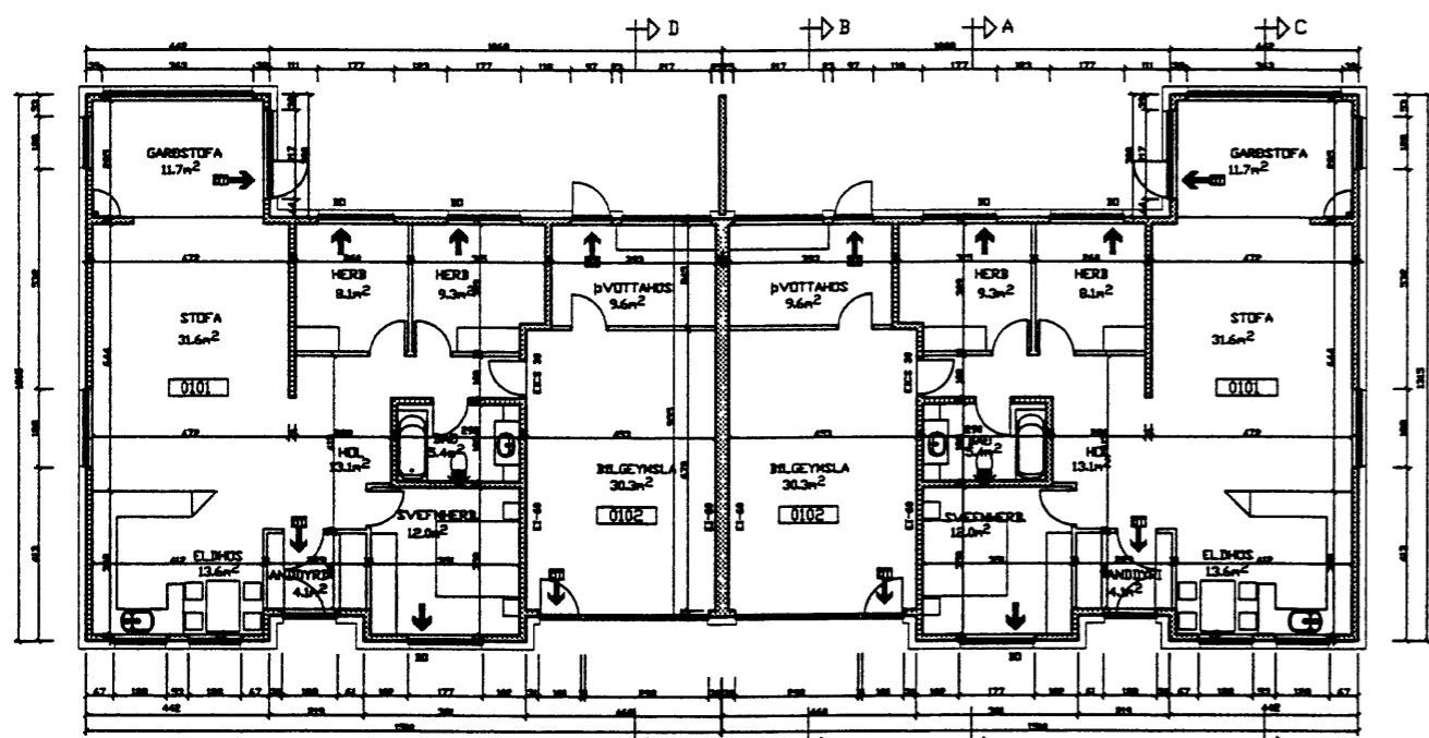
GRUNNMYND
