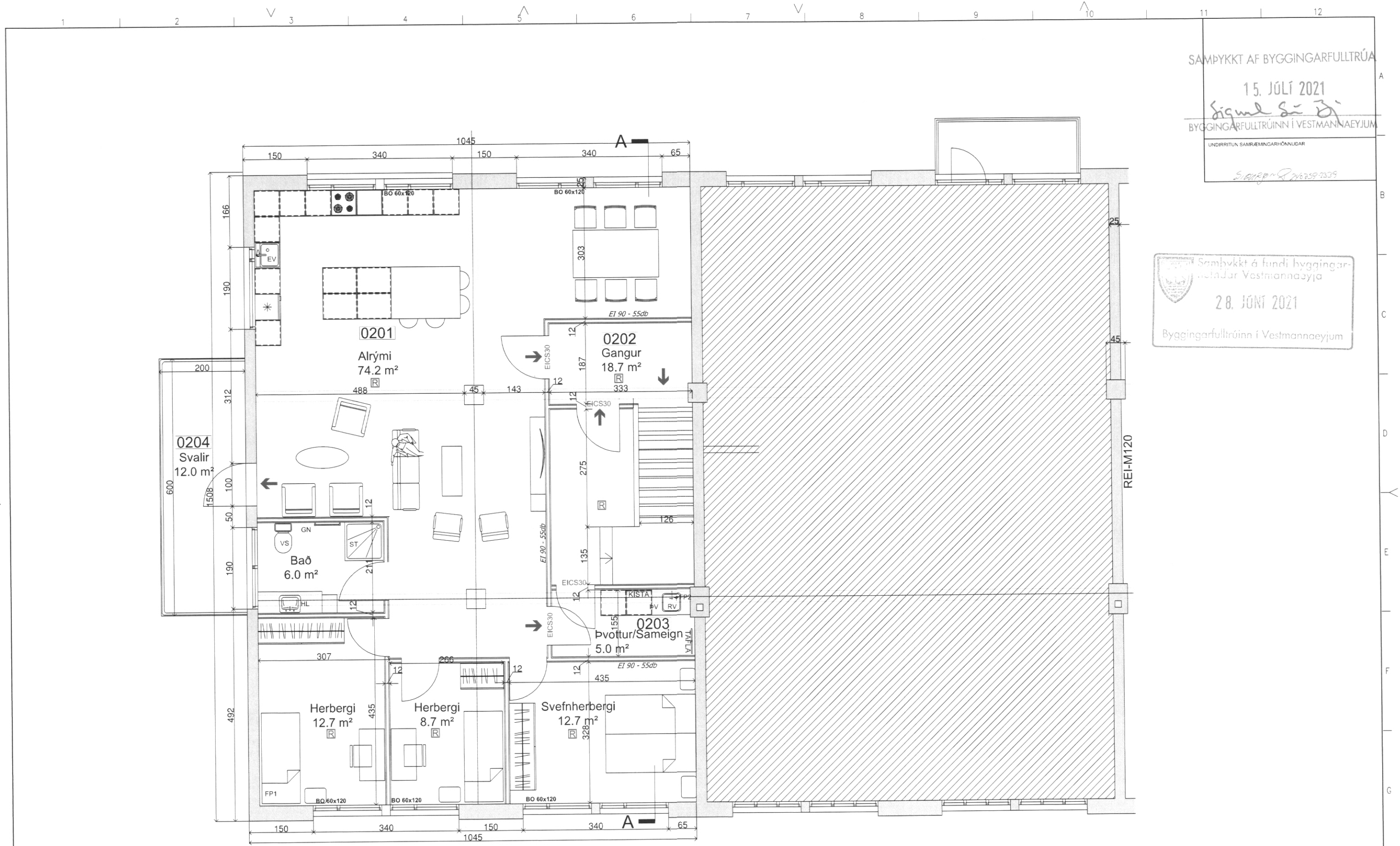
GRUNNMYND 2. HÆÐ
