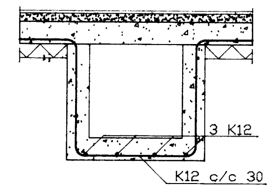
LAGNASTOKKUR UNDIR SALERNI M=1:20
