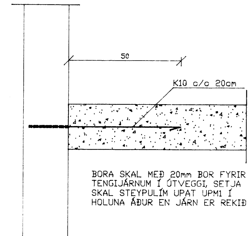
FRÁGANGUR ÚTVEGGJAR VIÐ ELÐRA HÚS M=1:10
