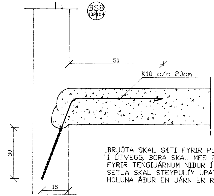
FRÁGANGUR ÚTVEGGJAR VIÐ ELÐRA HÚS M=1:10
