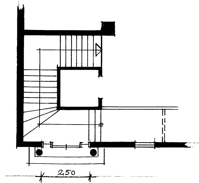
GRUNNMYND ANDDYRIS EFTIR BREYTINGU
