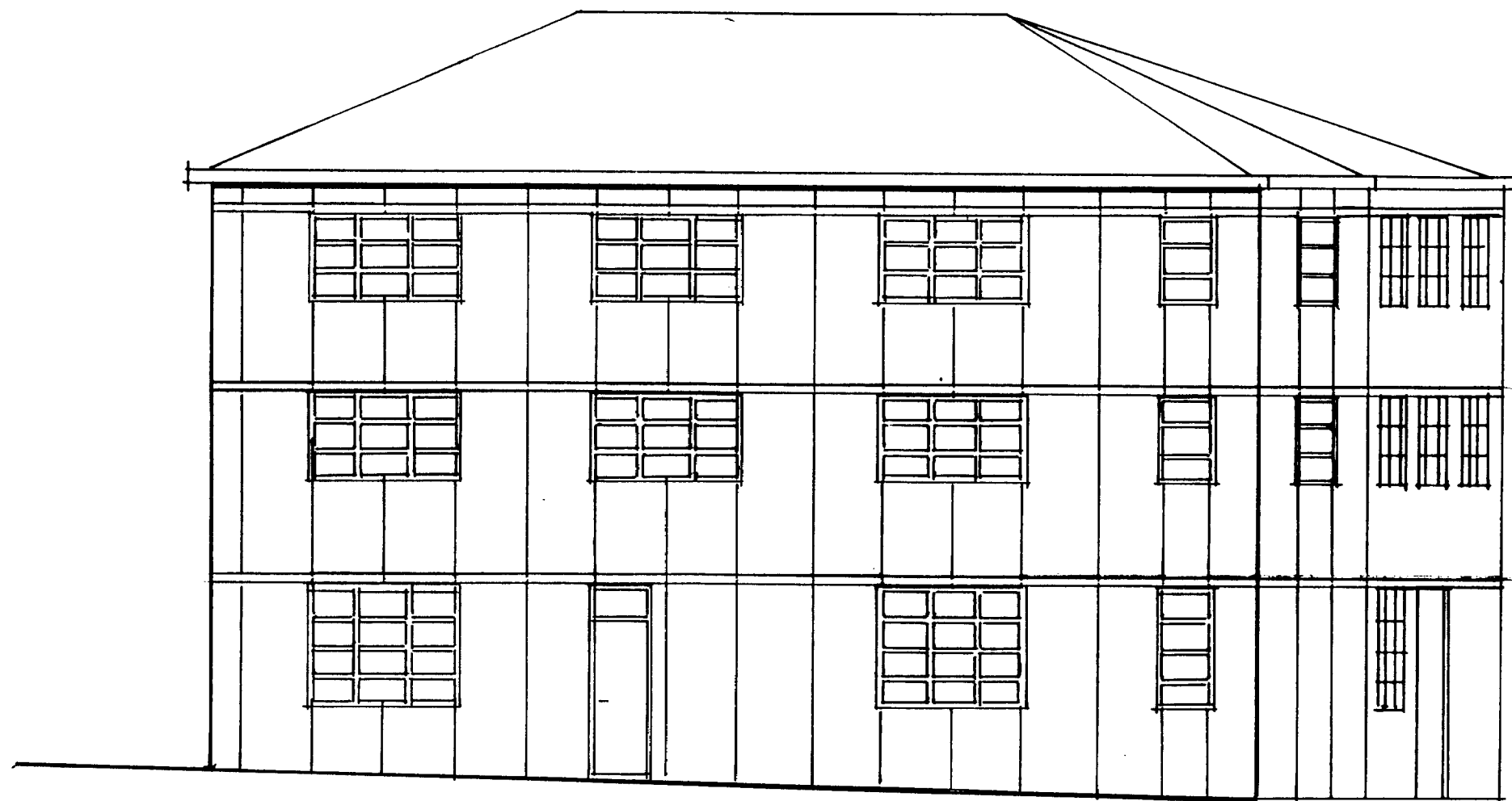
AUSTUR FYRIR BREYTINGU
