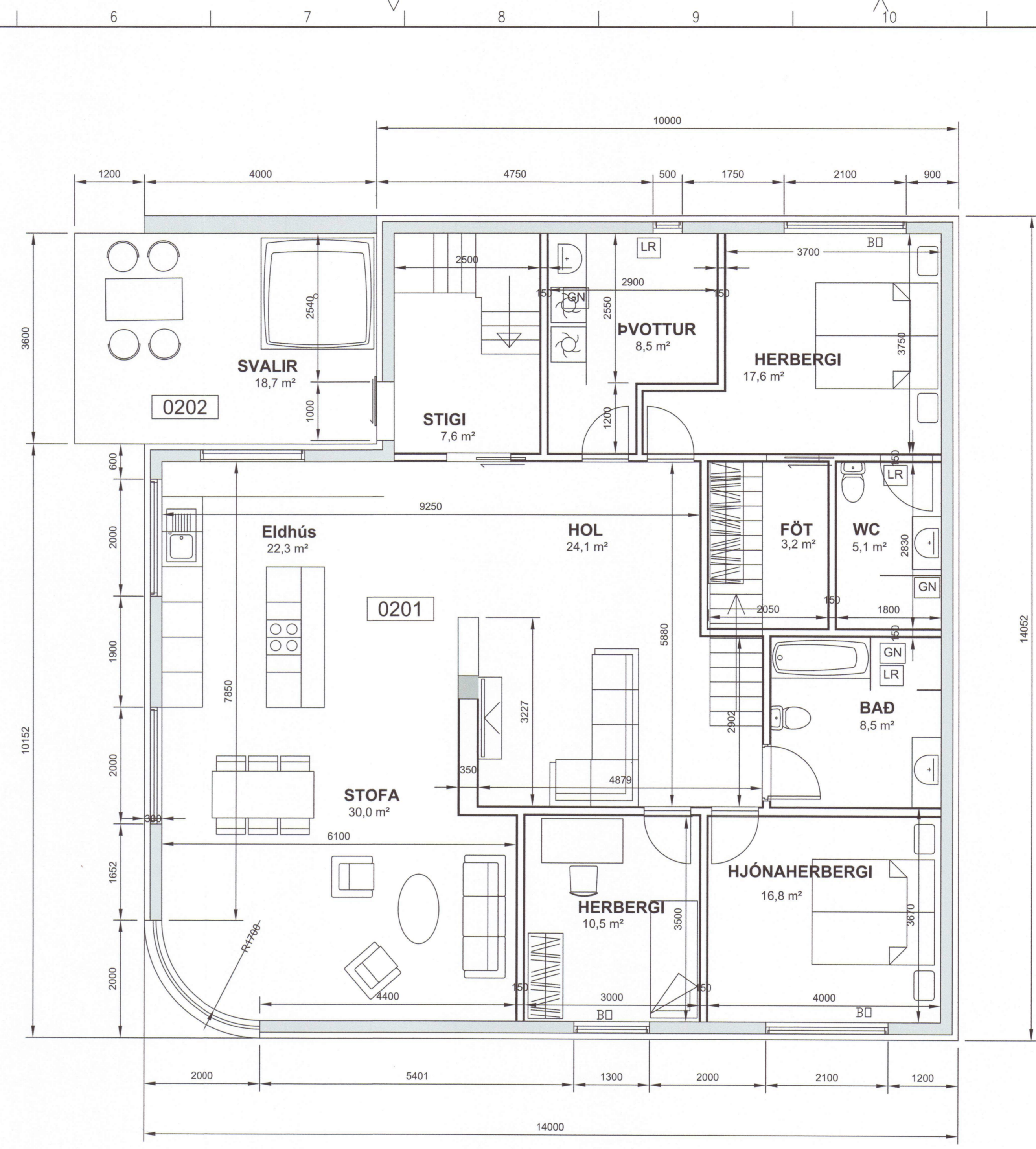
GRUNNMYND 2.HÆÐ 1:50
