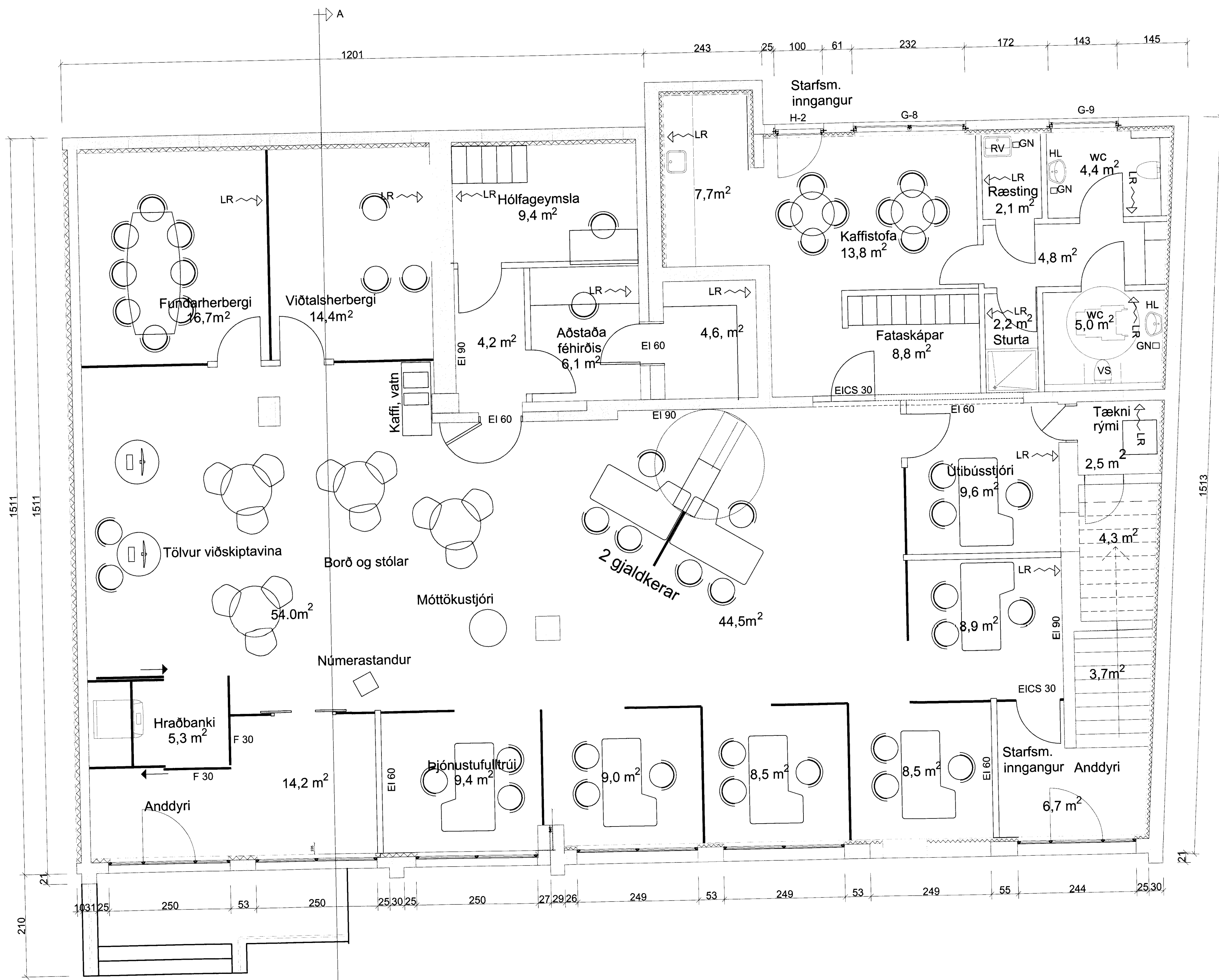
GRUNNMYND 1. HÆÐ M=1:100
