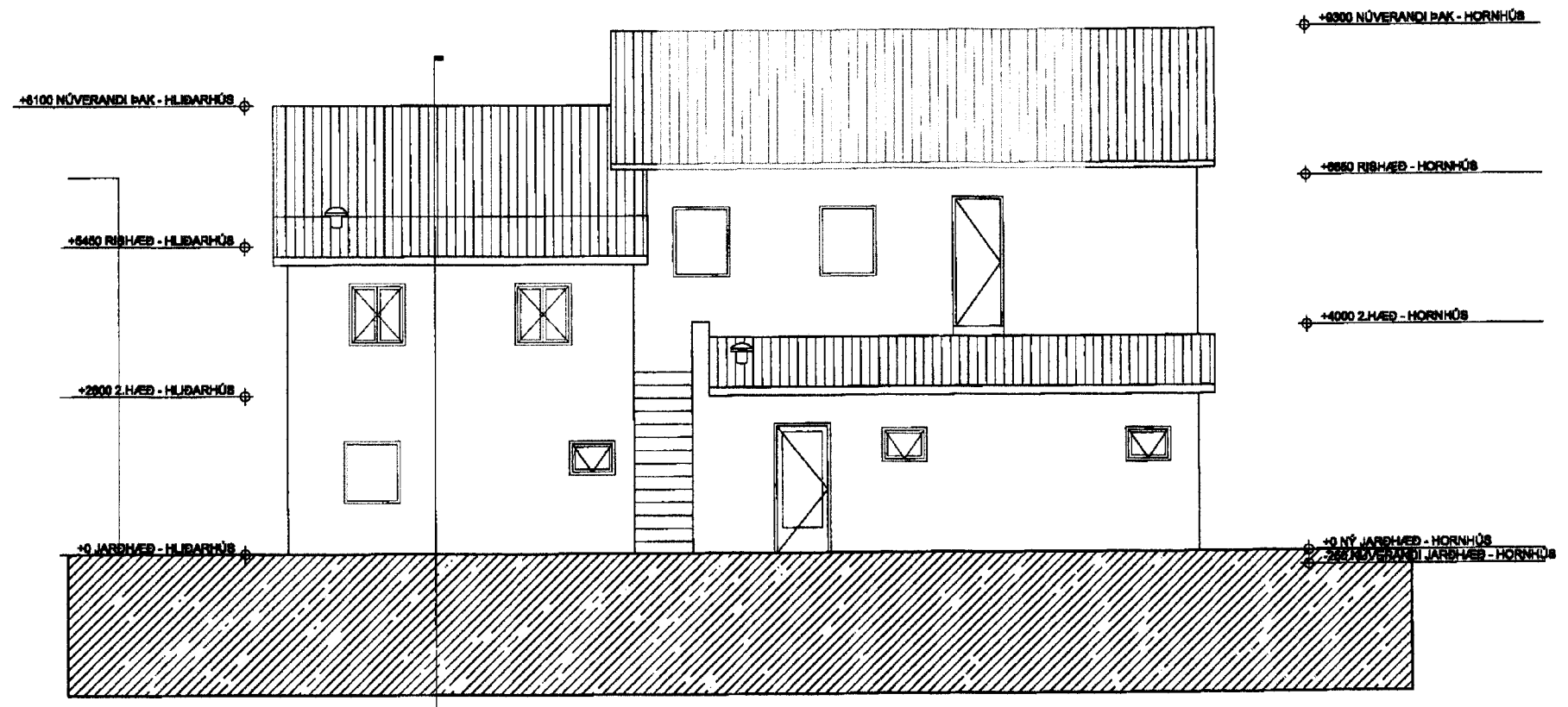
1 ÁSÝND AUSTURHLIÐ Scale: 1:100 @ A3
