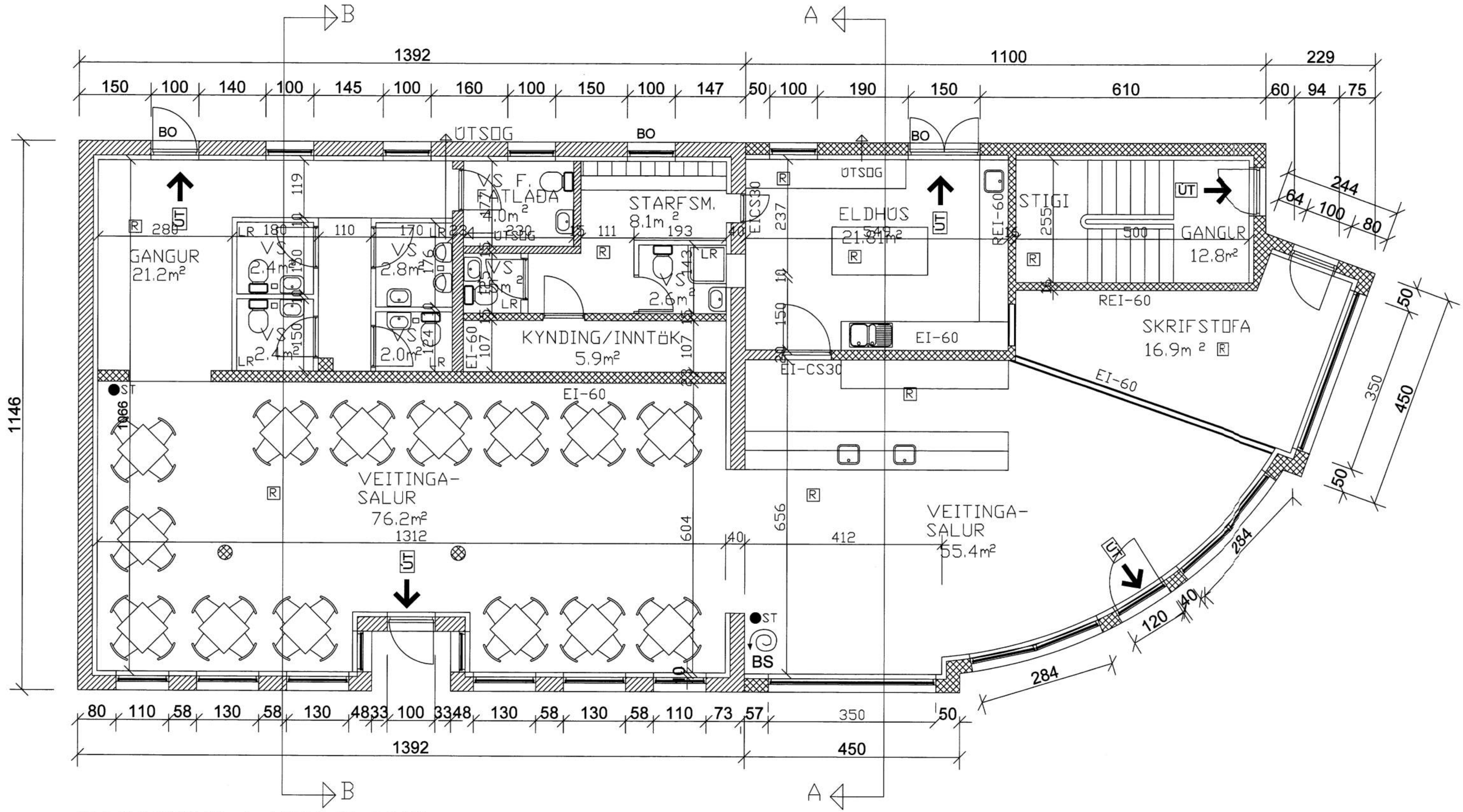
GRUNNMYND 1 HÆÐ M=1:100
