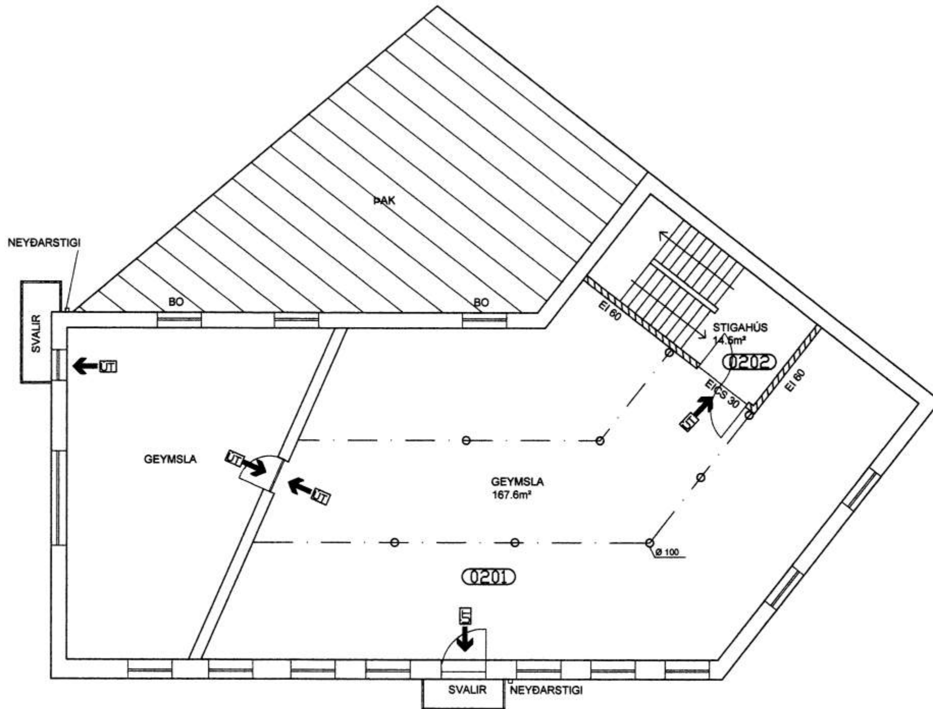
GRUNNMYND 2. HÆÐ M=1:50
